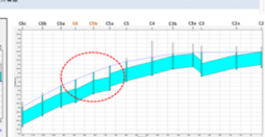
基地排水路動態檢核示意-人孔冒水
