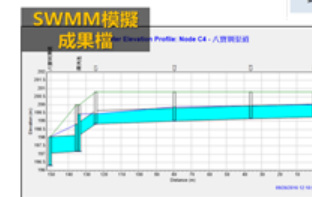
基地排水路動態檢核示意
