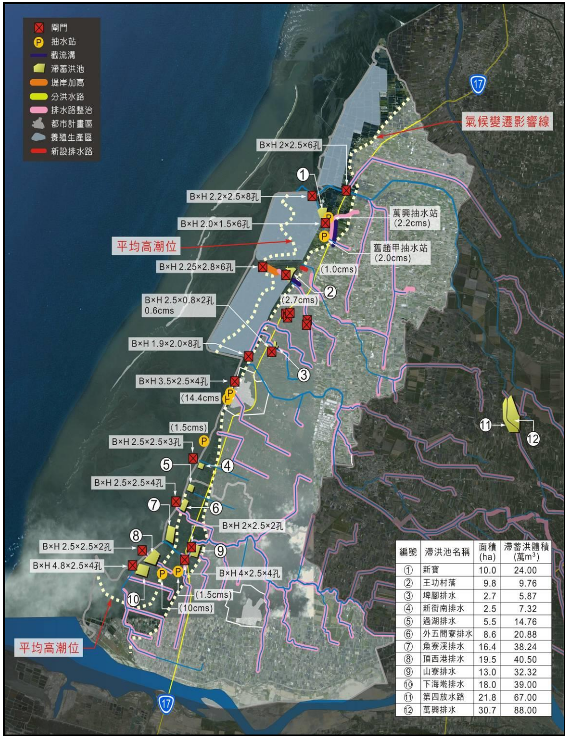
圖 5-2 彰化地區嚴重地層下陷地區綜合治水工程布置圖
