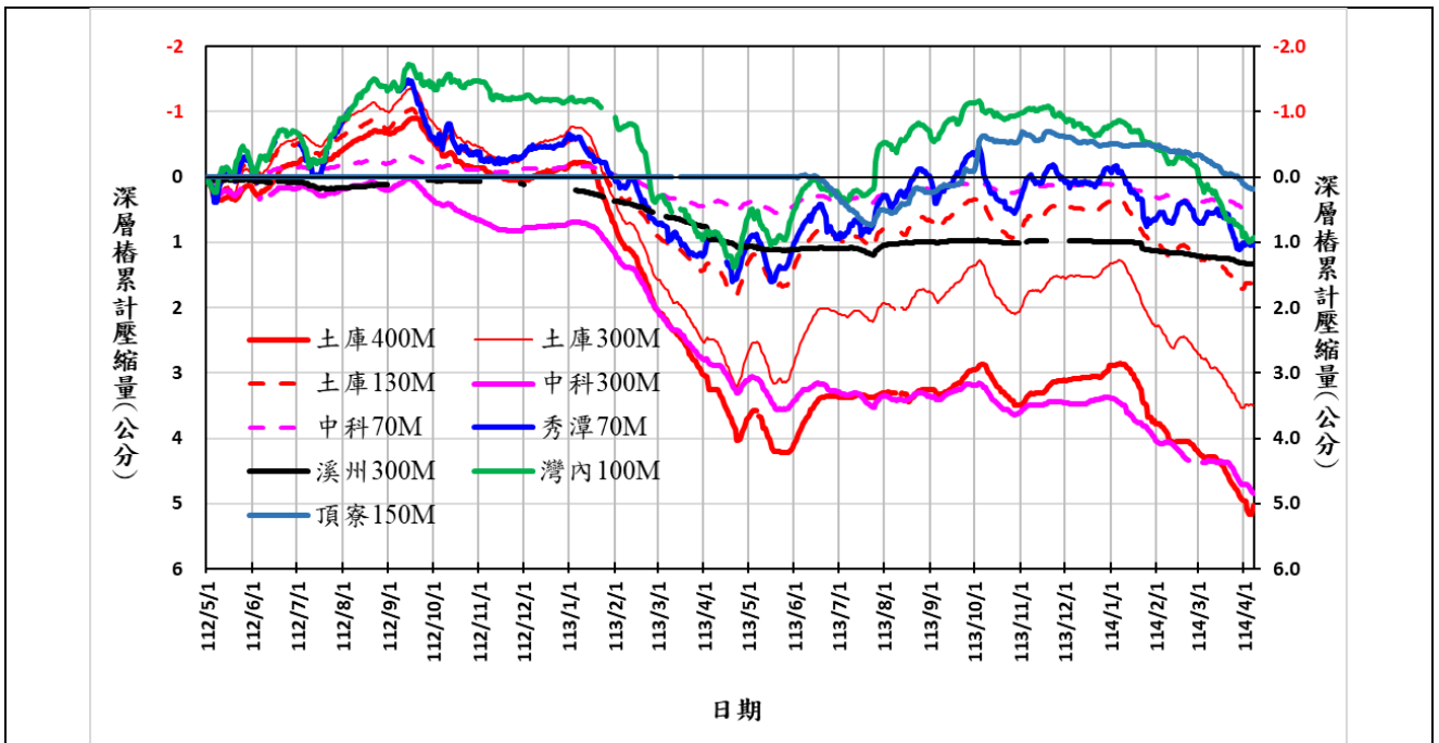
(A)彰雲嘉屏顯著下陷地區 112/5/1~114/3/31 期間的地層累計壓縮歷線圖
