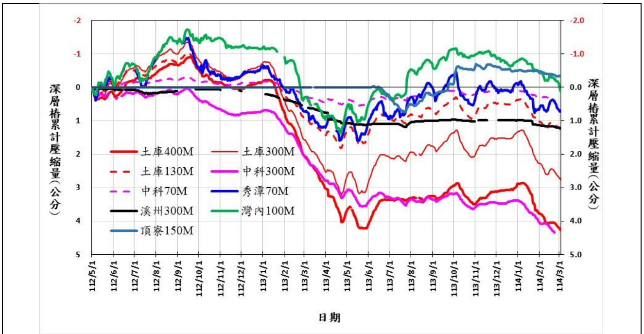
(A)彰雲嘉屏顯著下陷地區 112/5/1~114/2/28 期間的地層累計壓縮歷線圖
