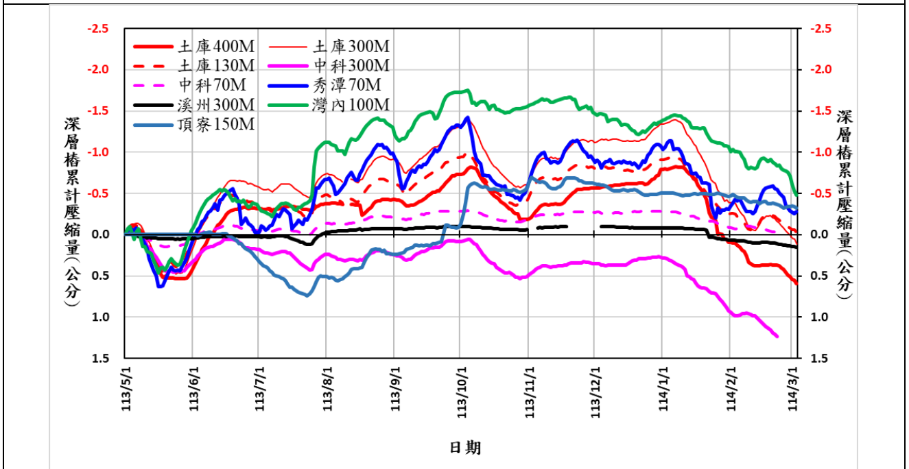
(B)彰雲嘉屏顯著下陷地區 113/5/1~114/2/28 期間的地層累計壓縮歷線圖
