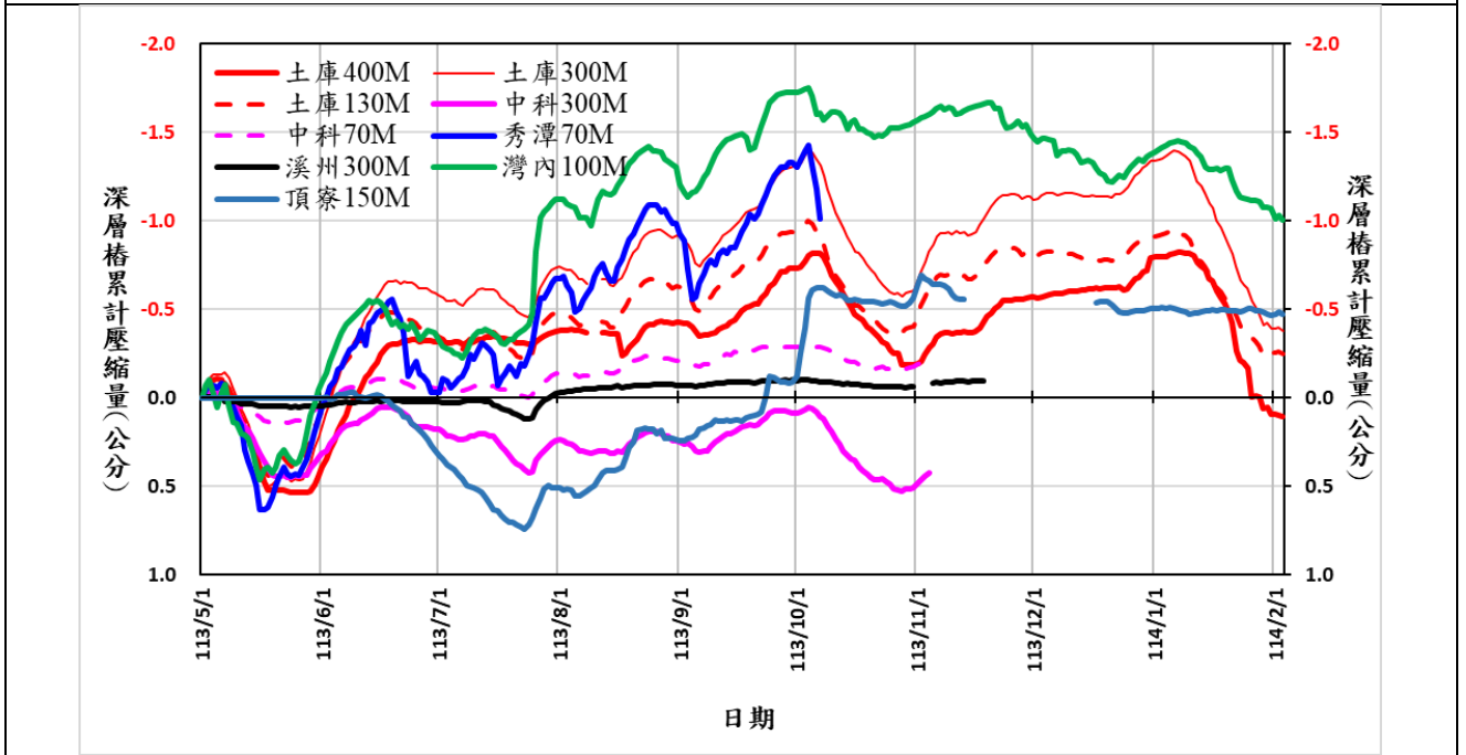
(B)彰雲嘉屏顯著下陷地區 113/5/1~114/1/31 期間的地層累計壓縮歷線圖
