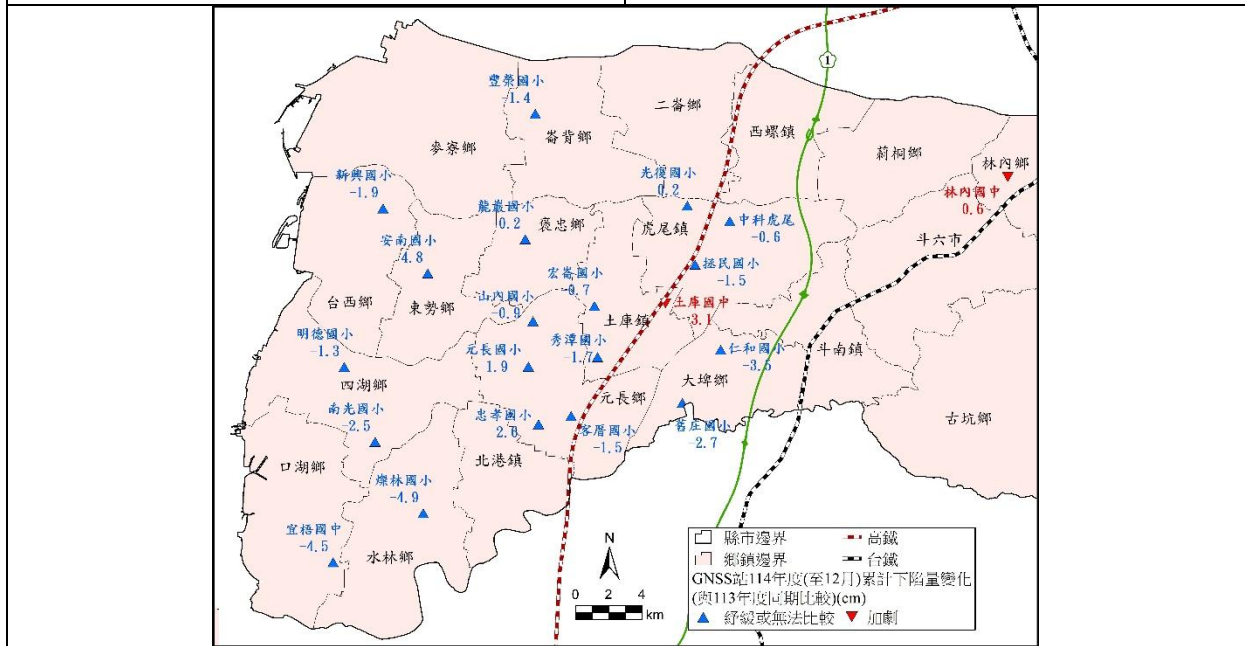
(C) 114 年 度 迄 今 (113/4~113/12) 雲 林 地 區 地 表 下 陷 情 勢 圖 (數 值 為 地 面 高 程 年 度 累 計 變 化 量, 正 值 表 下 陷、負 值 表 回 脹)
