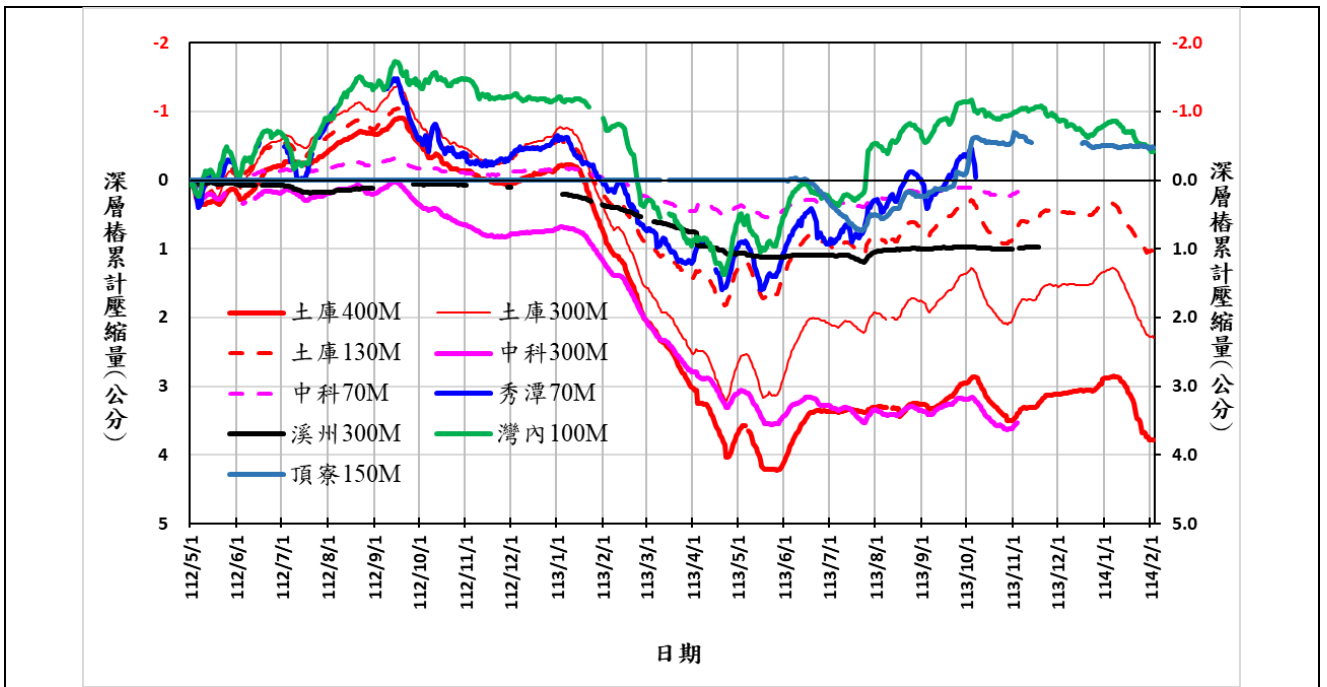
(A)彰雲嘉屏顯著下陷地區 112/5/1~114/1/31 期間的地層累計壓縮歷線圖
