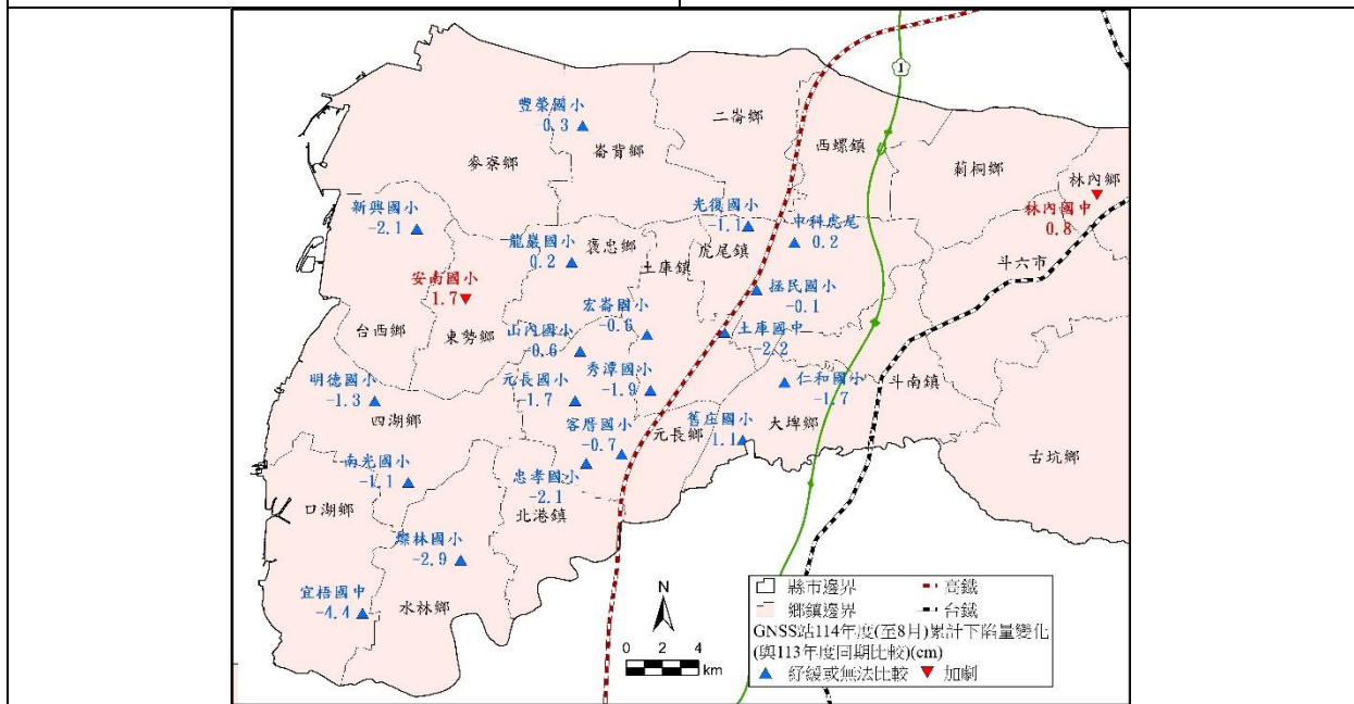
(C) 114 年度迄今(113/4~113/8)雲林地區地表下陷情勢圖 (數值為地面高程年度累計變化量, 正值表下陷、負值表回脹)
