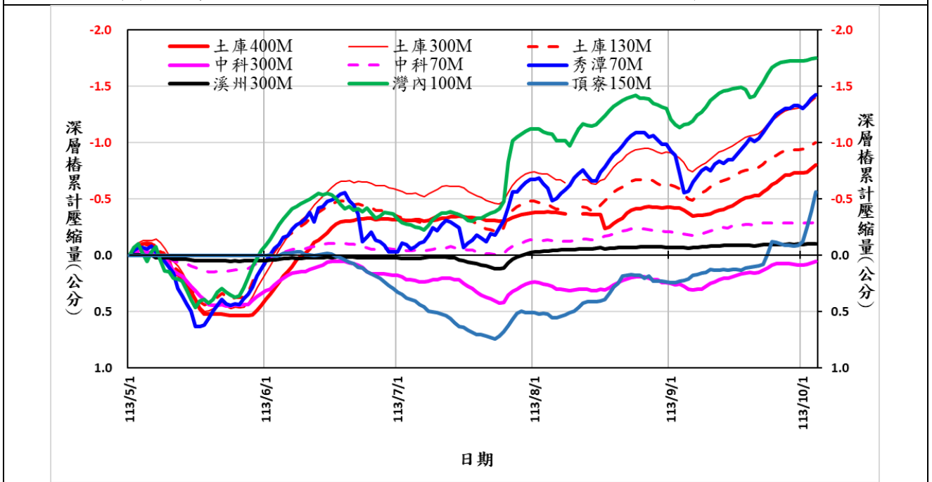
(B)彰雲嘉屏顯著下陷地區 113/5/1~113/9/30 期間的地層累計壓縮歷線圖
