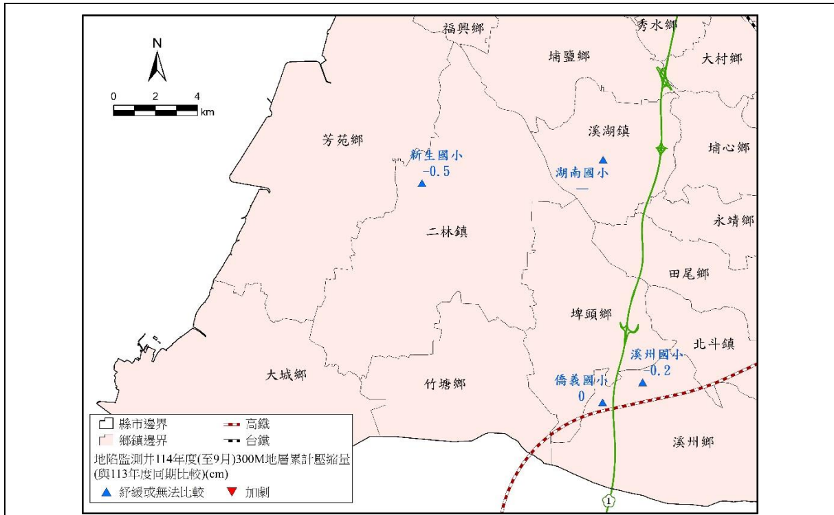
(A)彰化顯著下陷地區地表下 0~300 公尺地層本年度迄今(113/9)壓縮情勢圖 (圖中倒三角形表”顯著”壓縮；數值為地層厚度月變化量，正值表壓縮、負值表回脹)
