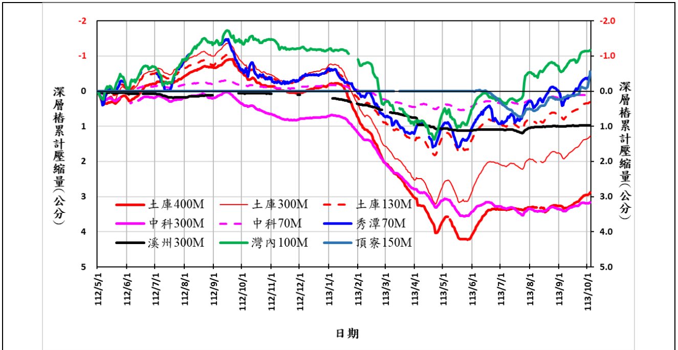
(A)彰雲嘉屏顯著下陷地區 112/5/1~113/9/30 期間的地層累計壓縮歷線圖
