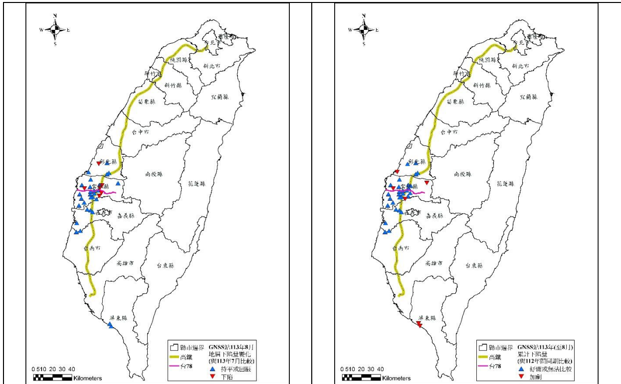
(B) 全臺最新年度(迄 113/8)地表下陷情勢與去年同期比較圖
