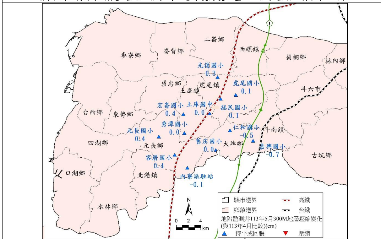
(B)雲林顯著下陷地區地表下0~300公尺地層 113 年 5 月壓縮情勢圖 (圖中倒三角形表壓縮”顯著”增加；數值為地層厚度月變化量，正值表壓縮、負值表回脹)
