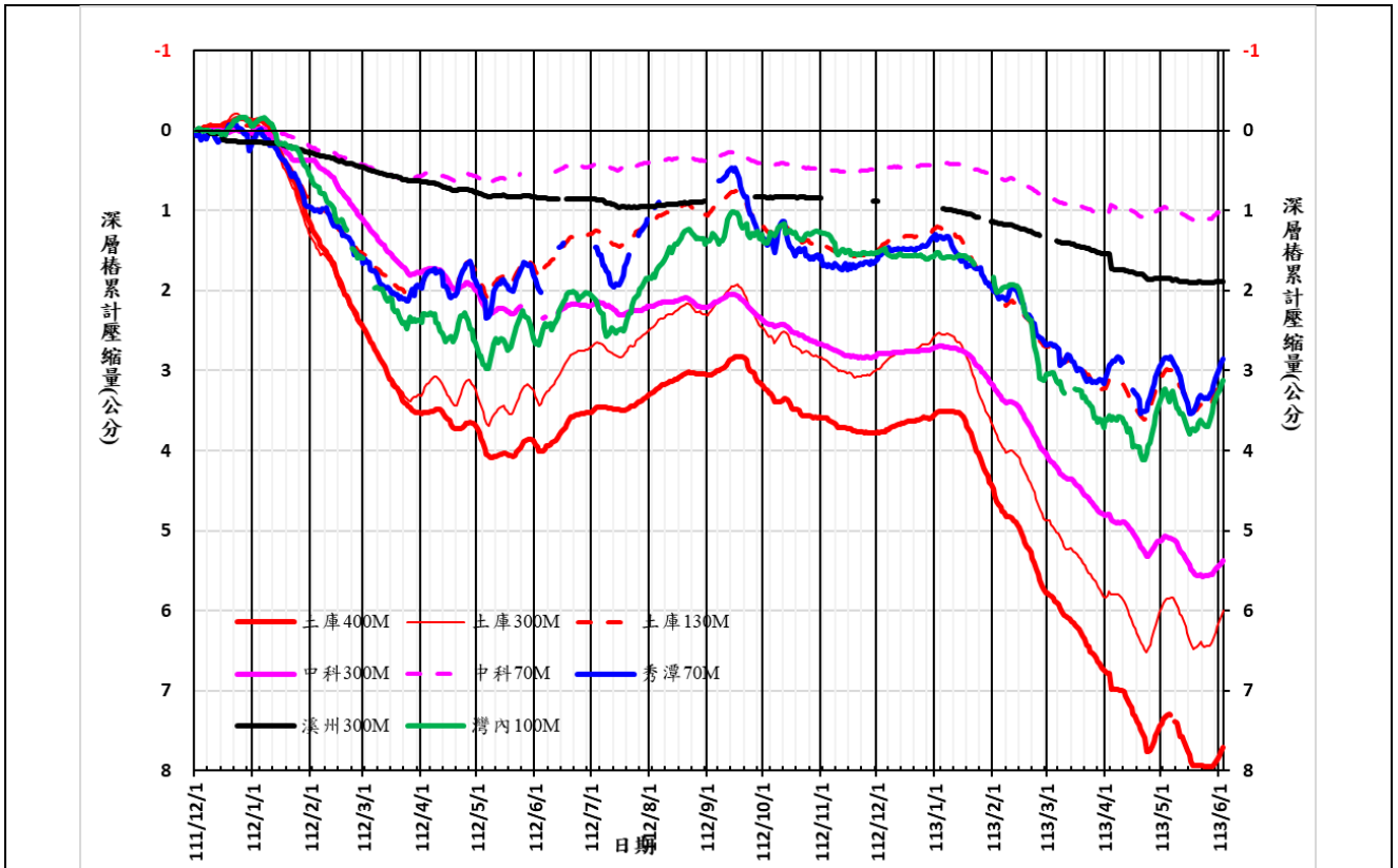
(A)彰雲嘉顯著下陷地區 111/12/1~113/5/31 期間的地層累計壓縮歷線圖
