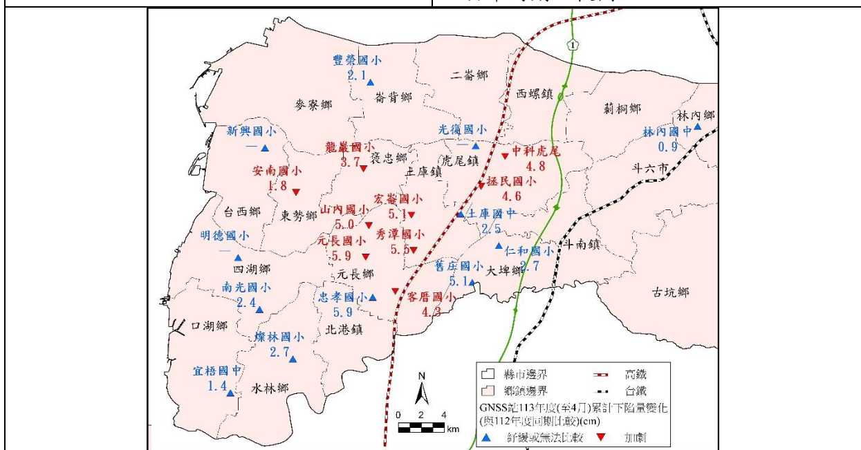
(C) 113 年 度 迄 今 (112/4~113/4) 雲 林 地 區 地 表 下 陷 情 勢 圖 (數 值 為 地 面 高 程 年 度 累 計 變 化 量, 正 值 表 下 陷、負 值 表 回 脹)
