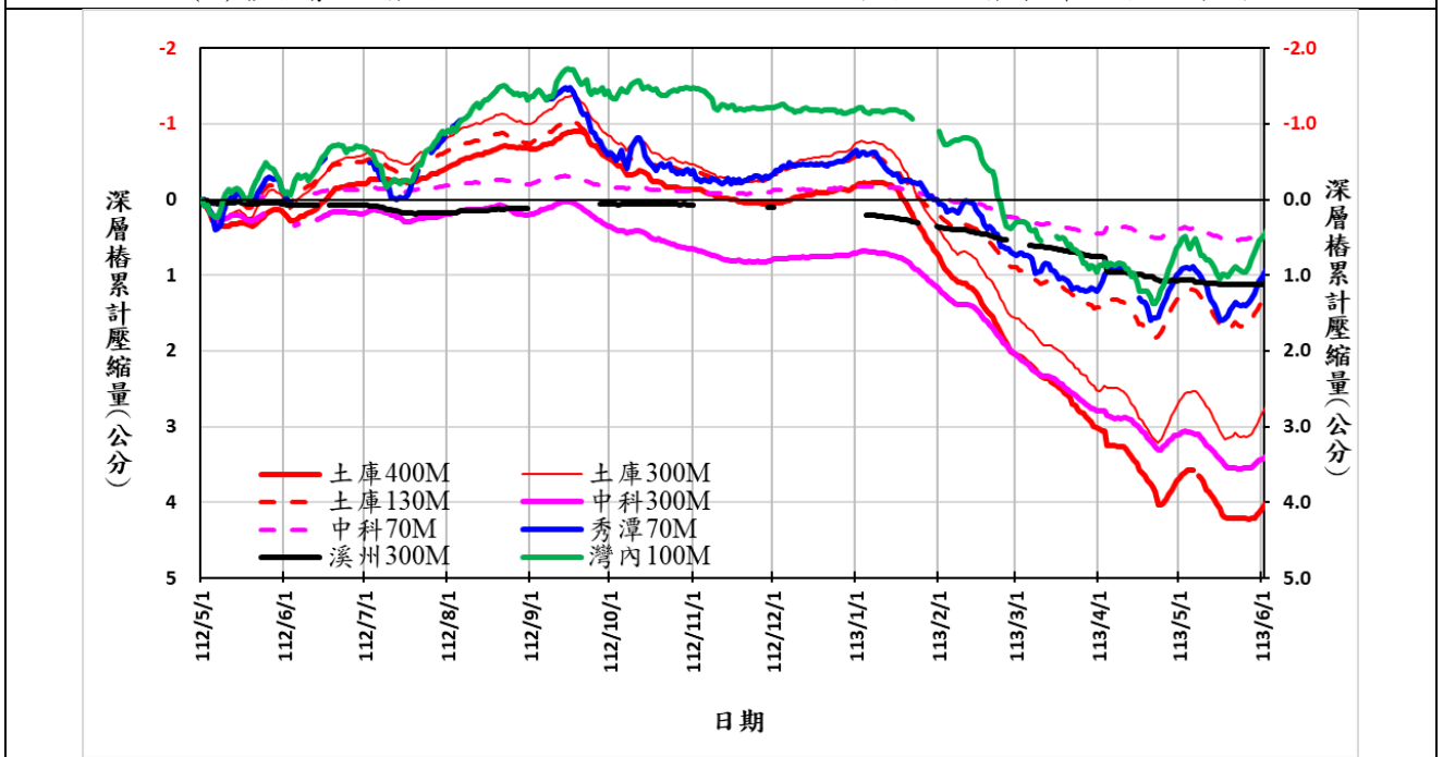
(B)彰雲嘉顯著下陷地區 112/5/1~113/5/31 期間的地層累計壓縮歷線圖
