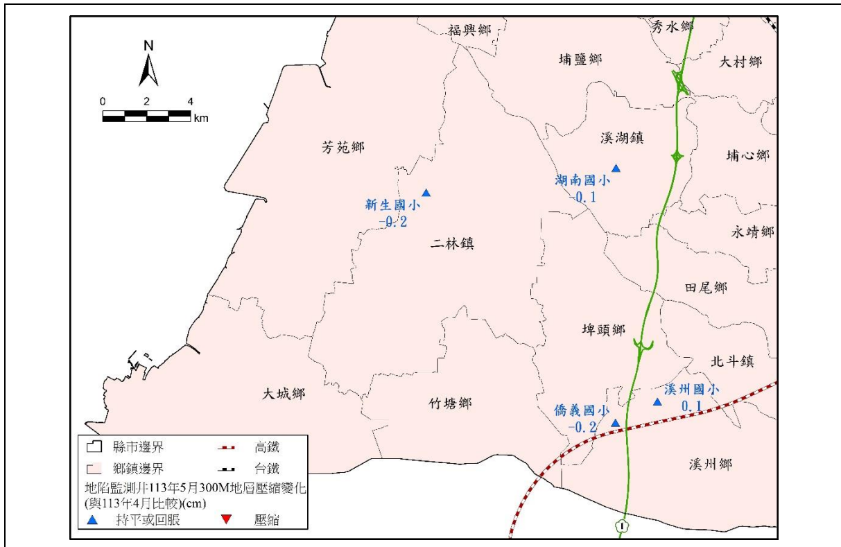
(A)彰化顯著下陷地區地表下0~300公尺地層 113 年 5 月壓縮情勢圖 (圖中倒三角形表”顯著”壓縮；數值為地層厚度月變化量，正值表壓縮、負值表回脹)
