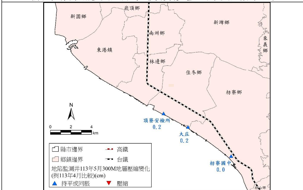
(D)屏東顯著下陷地區地表下0~300公尺地層113年5月壓縮情勢圖 (圖中倒三角形表壓縮”顯著”增加；數值為地層厚度月變化量，正值表壓縮、負值表回脹)
