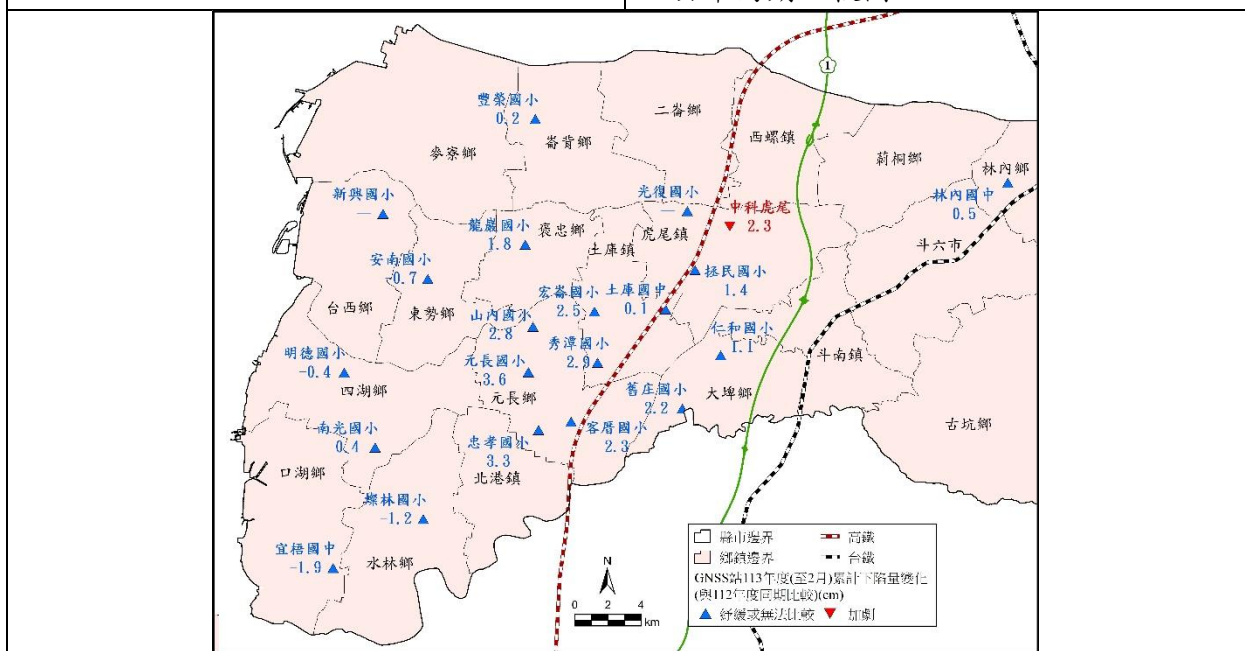
(C) 113年度迄今(112/4~113/2)雲林地區地表下陷情勢圖 (數值為地面高程年度累計變化量, 正值表下陷、負值表回脹)
