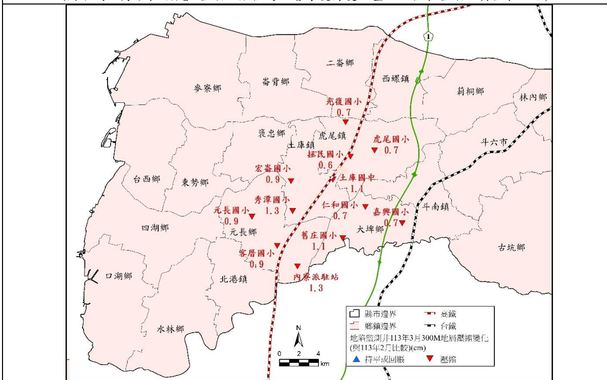
(B)雲林顯著下陷地區地表下0~300公尺地層 113 年 3 月壓縮情勢圖 (圖中倒三角形表壓縮”顯著”增加；數值為地層厚度月變化量，正值表壓縮、負值表回脹)
