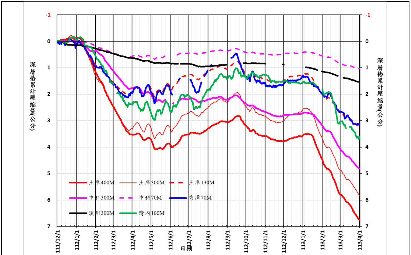
(A)彰雲嘉顯著下陷地區 111/12/1~113/3/31 期間的地層累計壓縮歷線圖
