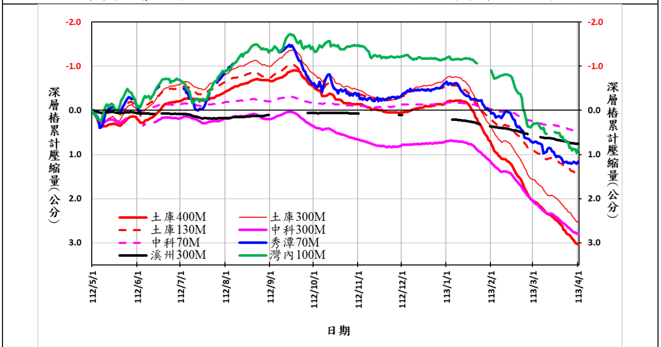
(B)彰雲嘉顯著下陷地區 112/5/1~113/3/31 期間的地層累計壓縮歷線圖
