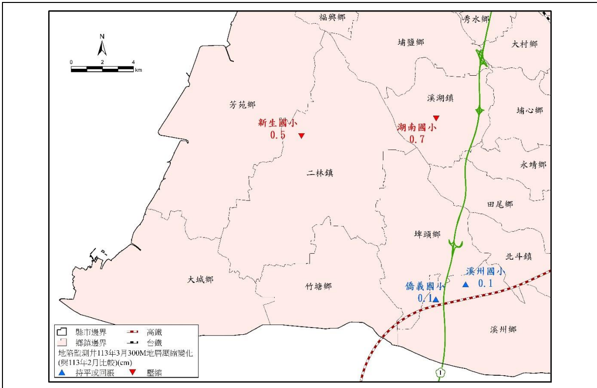
(A)彰化顯著下陷地區地表下0~300公尺地層 113 年 3 月壓縮情勢圖 (圖中倒三角形表”顯著”壓縮；數值為地層厚度月變化量，正值表壓縮、負值表回脹)
