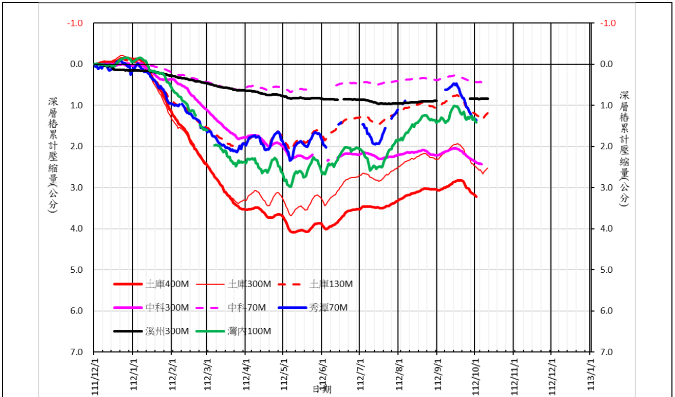
(A)彰雲嘉顯著下陷地區 111/12/1~112/9/30 期間的地層累計壓縮歷線圖
