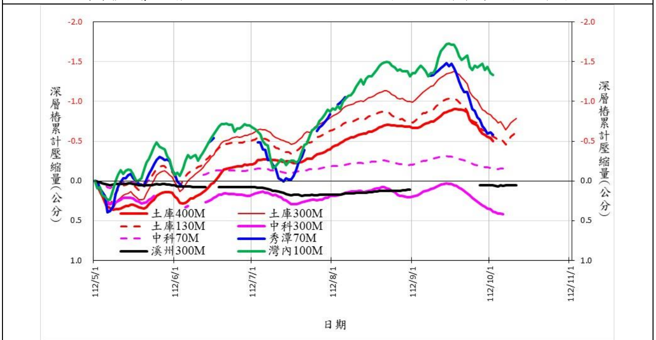
(B)彰雲嘉顯著下陷地區 112/5/1~113/9/30 期間的地層累計壓縮歷線圖
