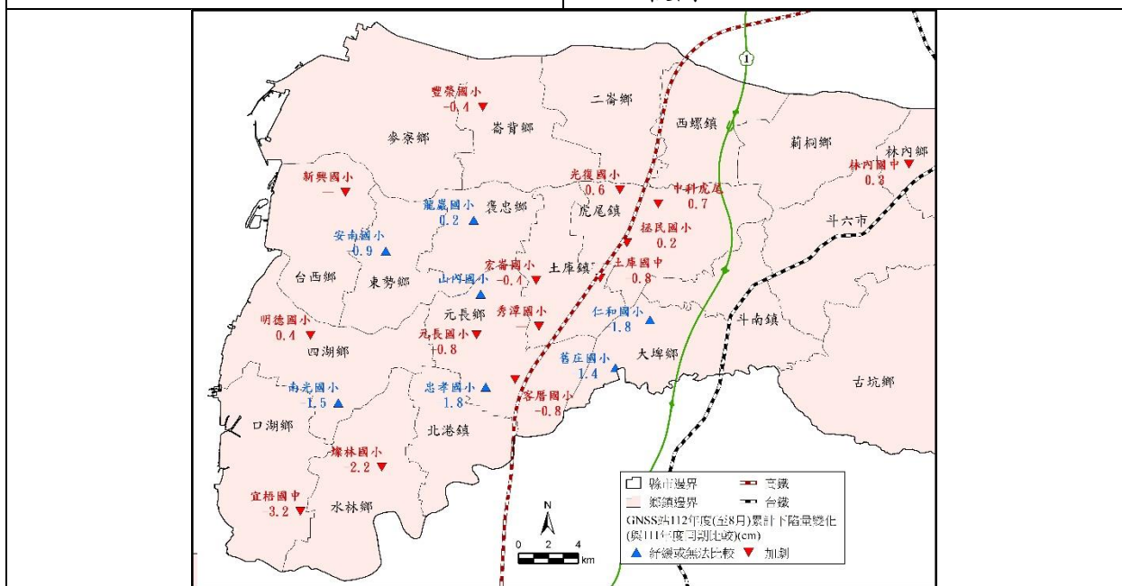
(C) 113 年 度 迄 今 (112/4~112/8) 雲 林 地 區 地 表 下 陷 情 勢 圖 (數 值 為 地 面 高 程 年 度 累 計 變 化 量, 正 值 表 下 陷、負 值 表 回 脹)
