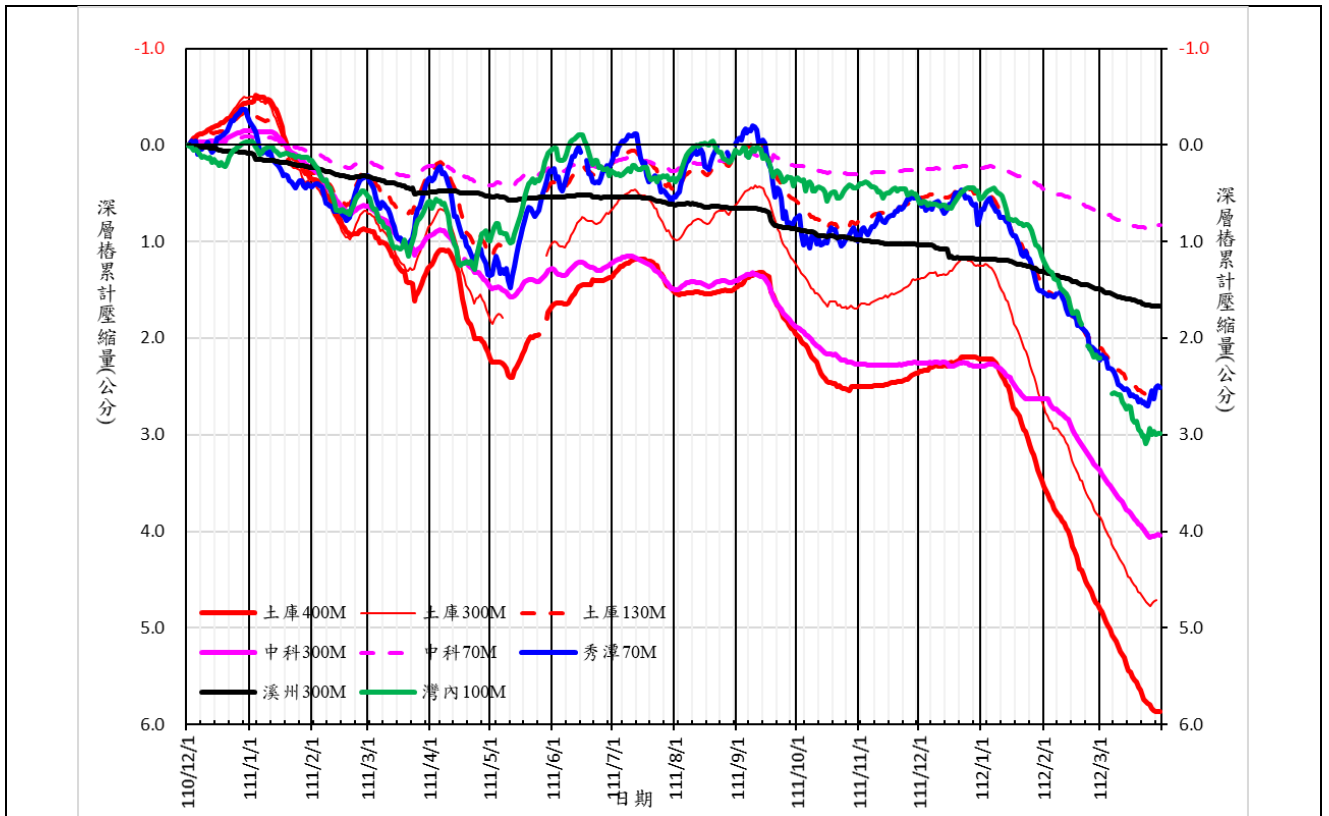
(A)彰雲嘉顯著下陷地區 110/12/1~112/3/31 期間的地層累計壓縮歷線圖
