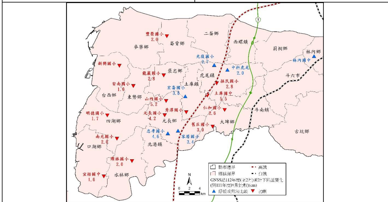
(C) 112 年 度 迄 今 (111/4~112/2) 雲 林 地 區 地 表 下 陷 情 勢 圖
