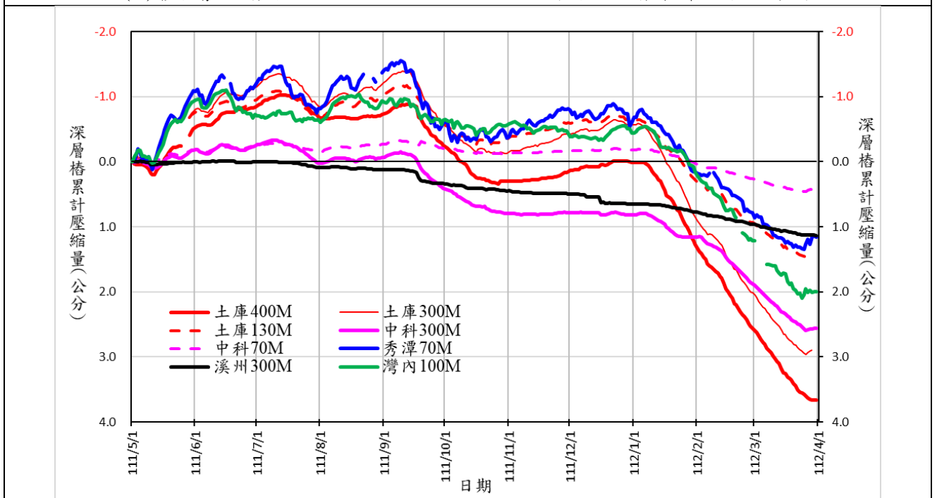
(B)彰雲嘉顯著下陷地區 111/5/1~112/3/31 期間的地層累計壓縮歷線圖
