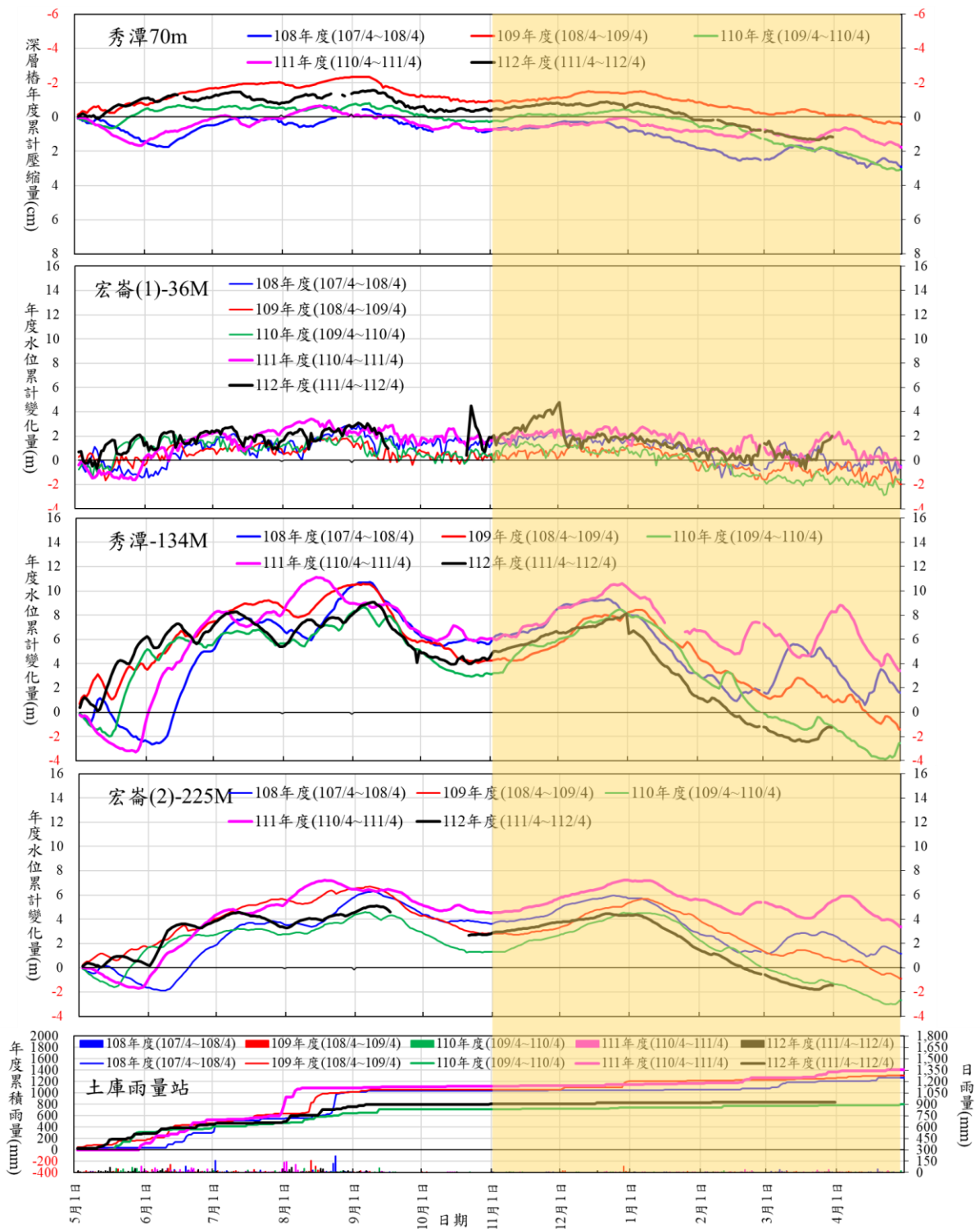
圖 10 雲林土庫秀潭地區降雨、地下水水位與地層壓縮變化情勢
