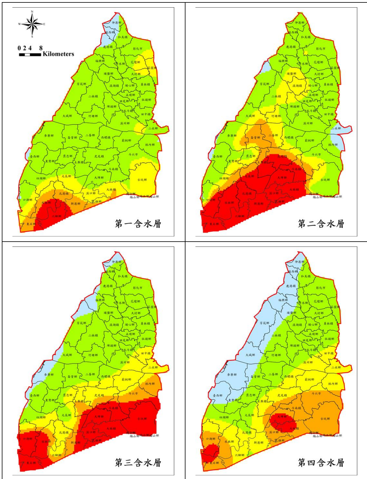
註：1.資料來源：臺灣水文環境通訊 112 年 2 月刊。 2.藍色表上升超過 1 公尺(含)以上，淺藍色表上升 0~1 公尺，綠色表下降 0~1 公尺，黃色表下降 1(含)~2 公尺，橙色表下降 2~3 公尺，紅色表下降超過 3 公尺(含)以上。
