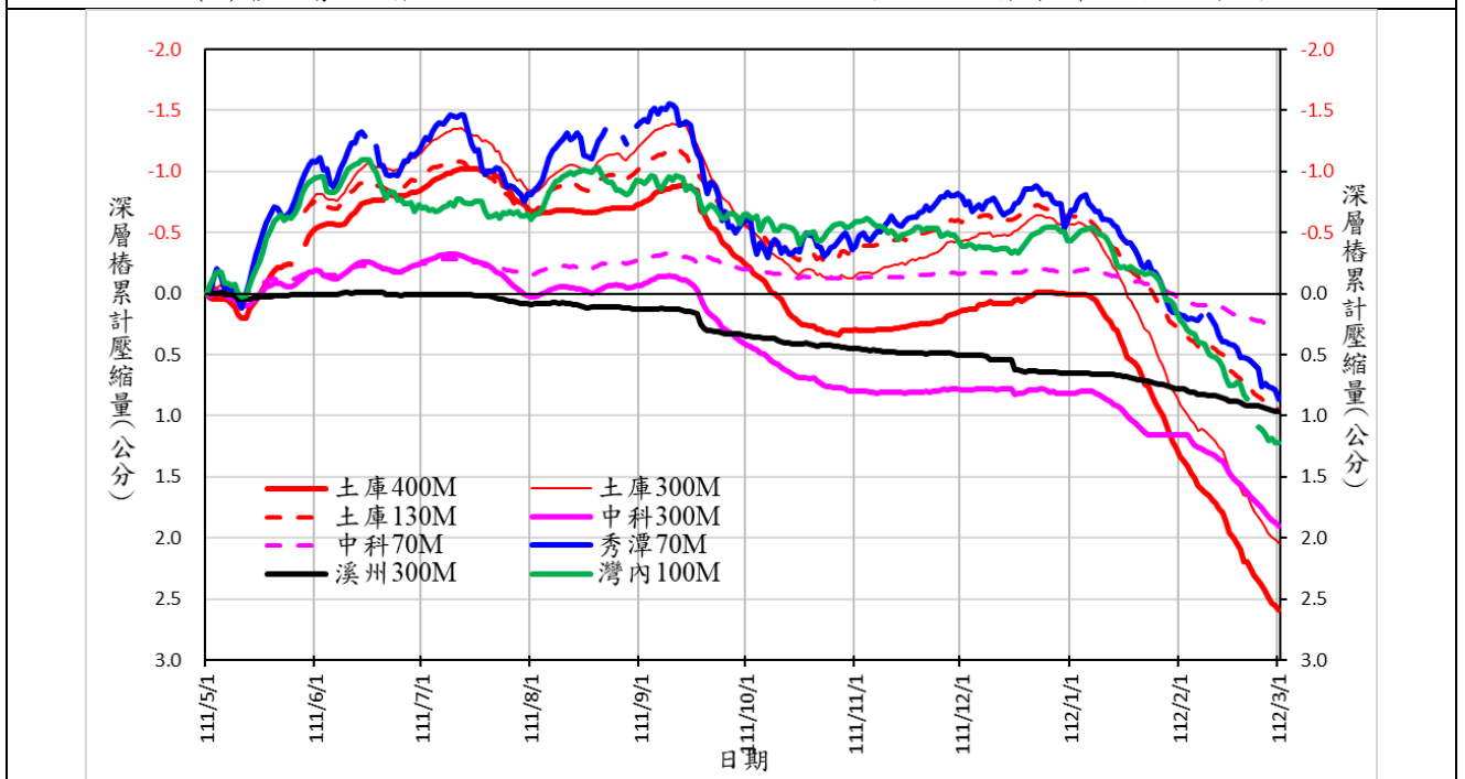
(B)彰雲嘉顯著下陷地區 111/5/1~112/2/28 期間的地層累計壓縮歷線圖
