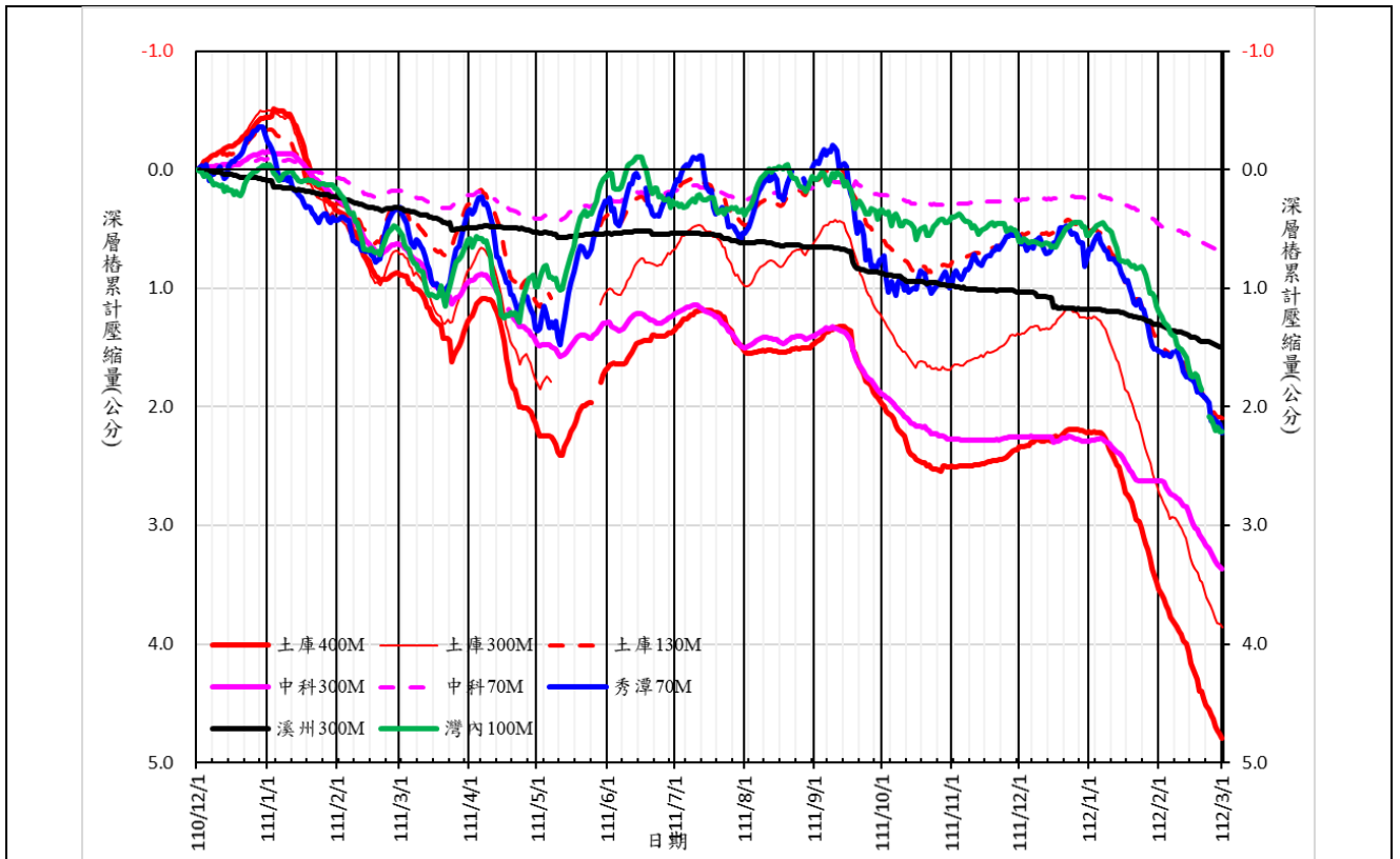
(A)彰雲嘉顯著下陷地區 110/12/1~112/2/28 期間的地層累計壓縮歷線圖
