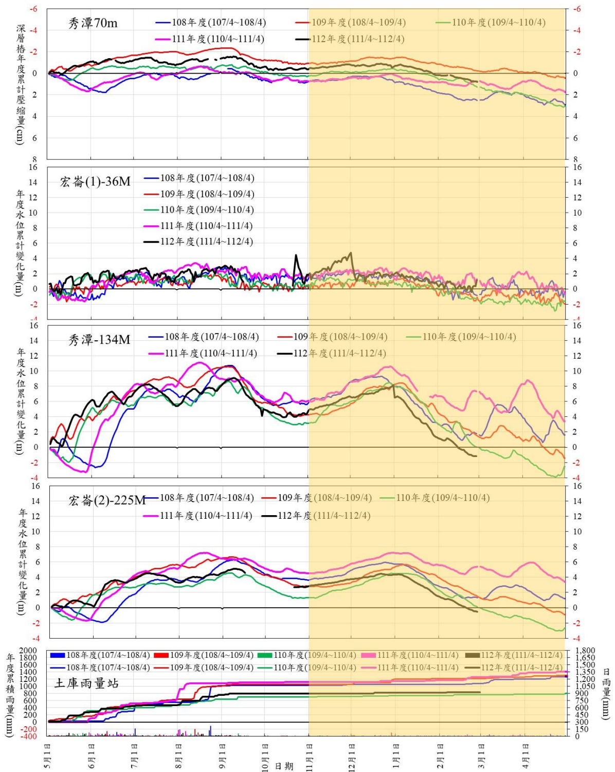
圖 9 雲林土庫秀潭地區降雨、地下水水位與地層壓縮變化情勢
