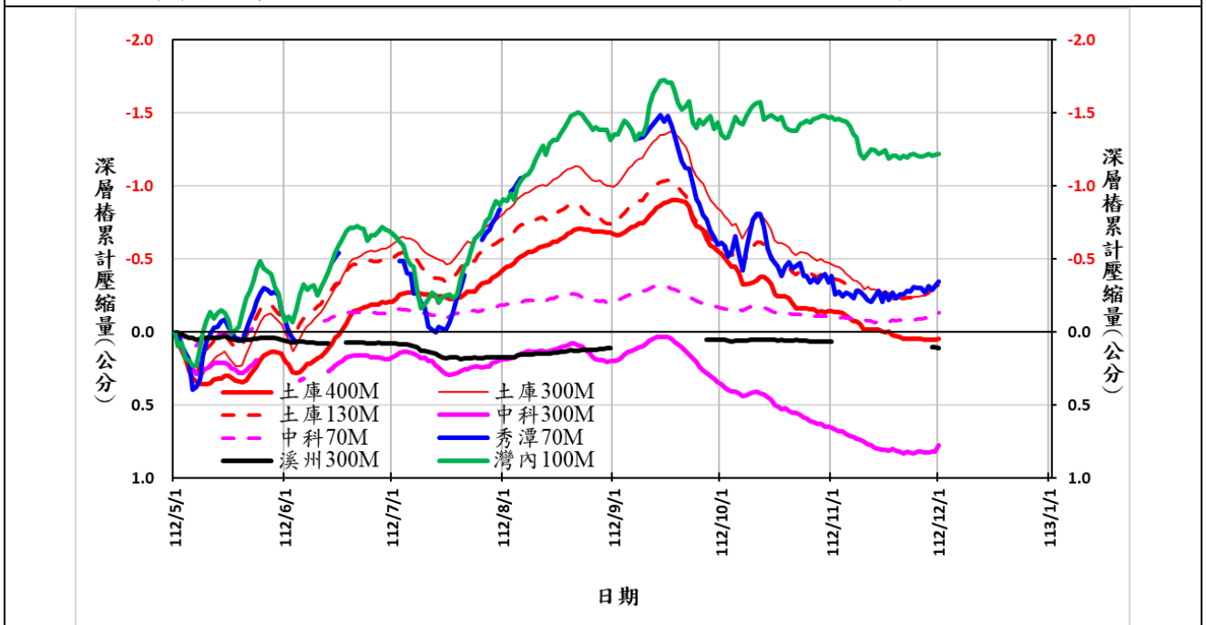
(B)彰雲嘉顯著下陷地區 112/5/1~113/11/30 期間的地層累計壓縮歷線圖
