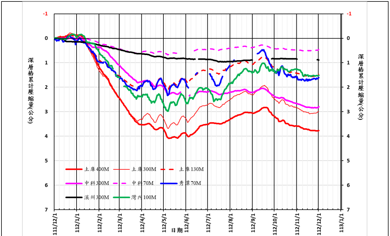
(A)彰雲嘉顯著下陷地區 111/12/1~112/11/30 期間的地層累計壓縮歷線圖
