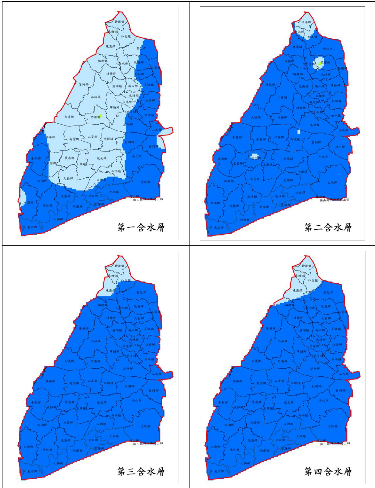
註：1.資料來源：臺灣水文環境通訊 111 年 3 月刊。 2.藍色表上升超過 1 公尺(含)以上，淺藍色表上升 0~1 公尺，綠色表下降 0~1 公尺，黃色表下降 1(含)~2 公尺，橙色表下降 2~3 公尺，紅色表下降超過 3 公尺(含)以上。
