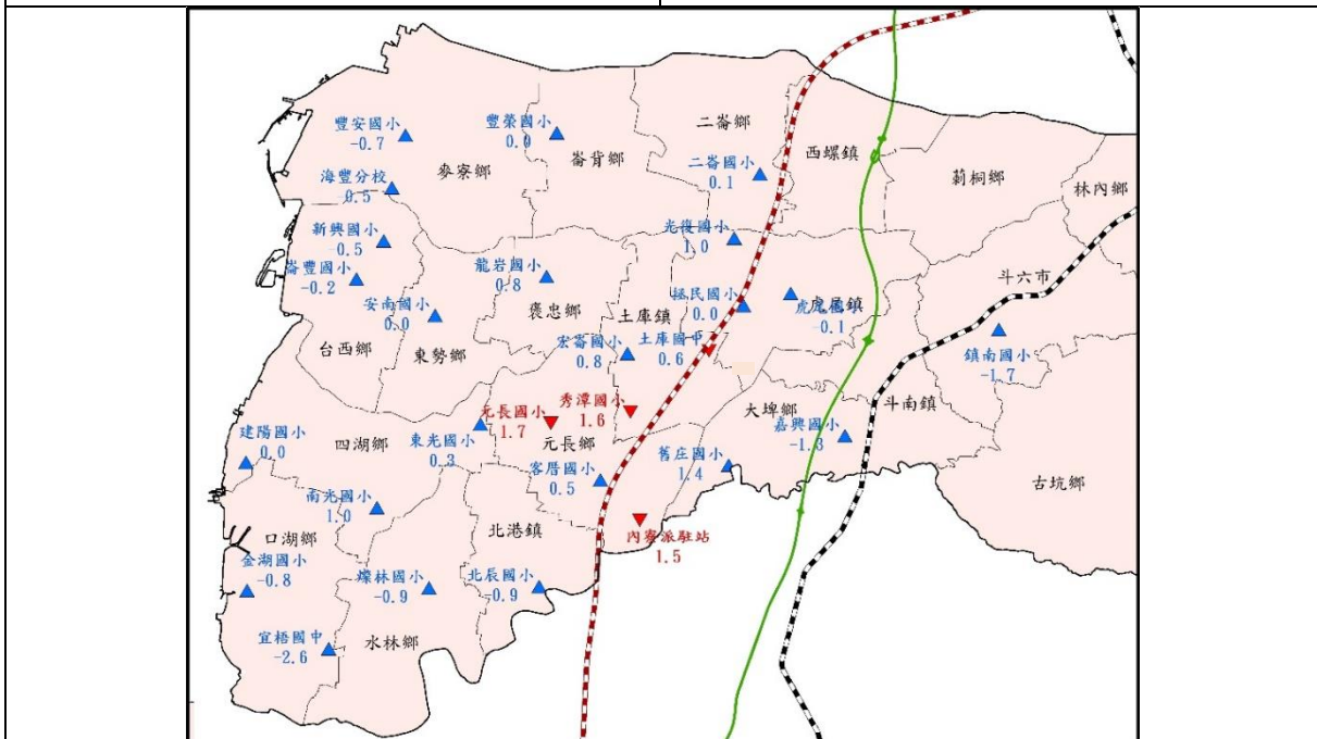
(C) 111 年度迄今(110/4~110/12)雲林地區地表下 0~300 公尺地層壓縮情勢圖 (圖中數值為地層厚度年度累計變化量，正值表壓縮、負值表回脹)
