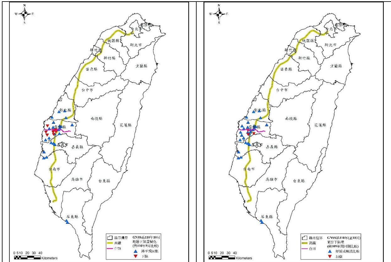
(B) 全 臺 最 新 年 度 (迄 110/10 止) 地 表 下 陷 情 勢 與 去 年 同 期 比 較 圖
