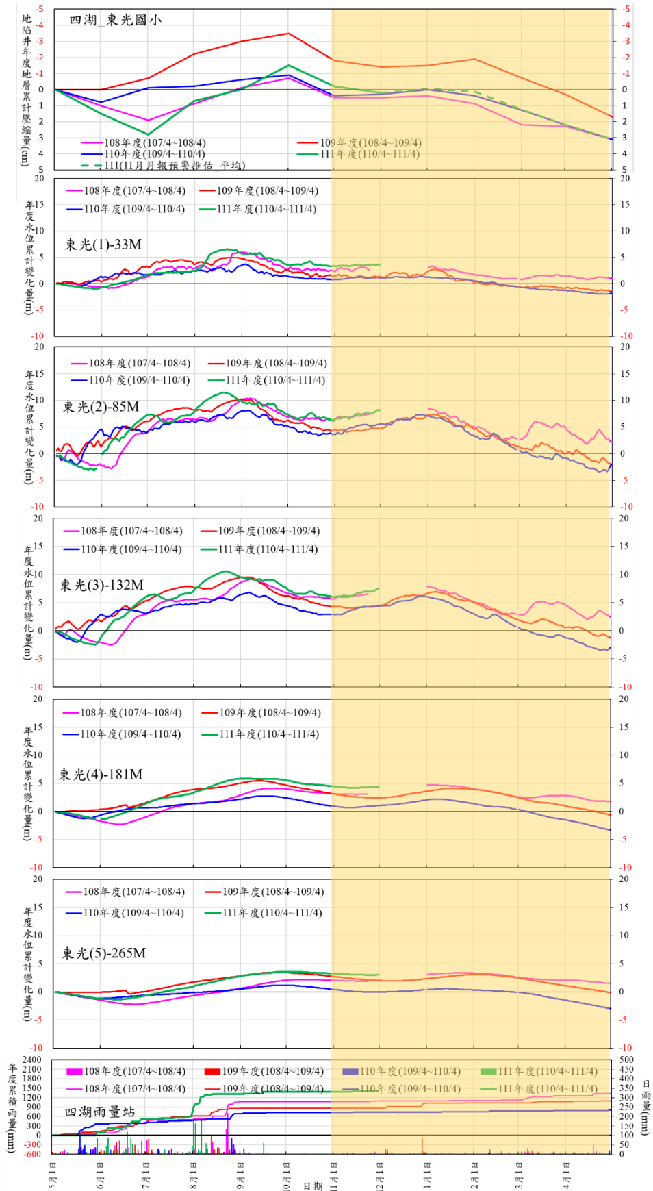
圖 7 雲林四湖地區降雨、地下水水位與地層壓縮變化情勢
