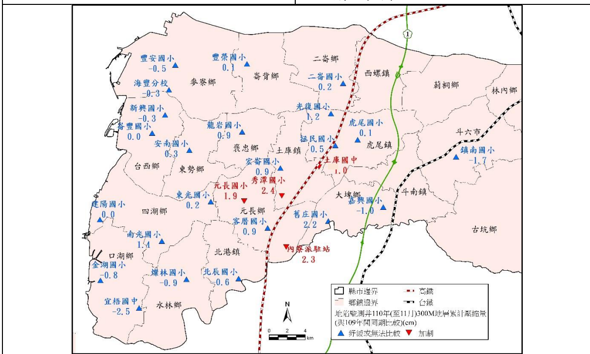
(C) 111 年度迄今(110/4~110/11)雲林地區地表下 0~300 公尺地層壓縮情勢圖
