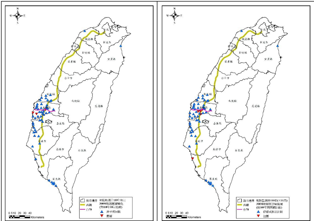
(A) 本月(110/11)全臺地表下 0~300 公尺地層壓縮情勢圖
