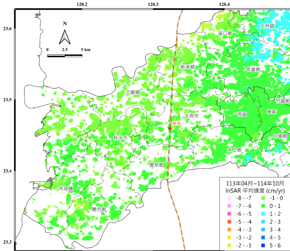
圖 6 嘉義地區 113 年 4 月~114 年 10 月之位移速度場
