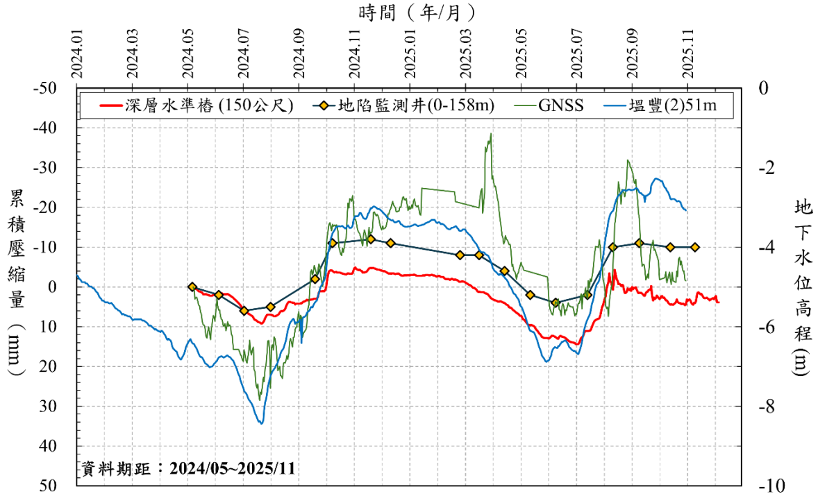
圖 5 屏東縣頂寮安檢所 106/7~114/10 監測成果分析圖
