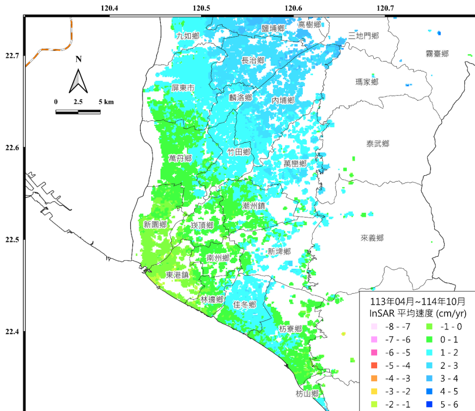
圖 7 屏東地區 113 年 4 月~114 年 10 月之位移速度場
