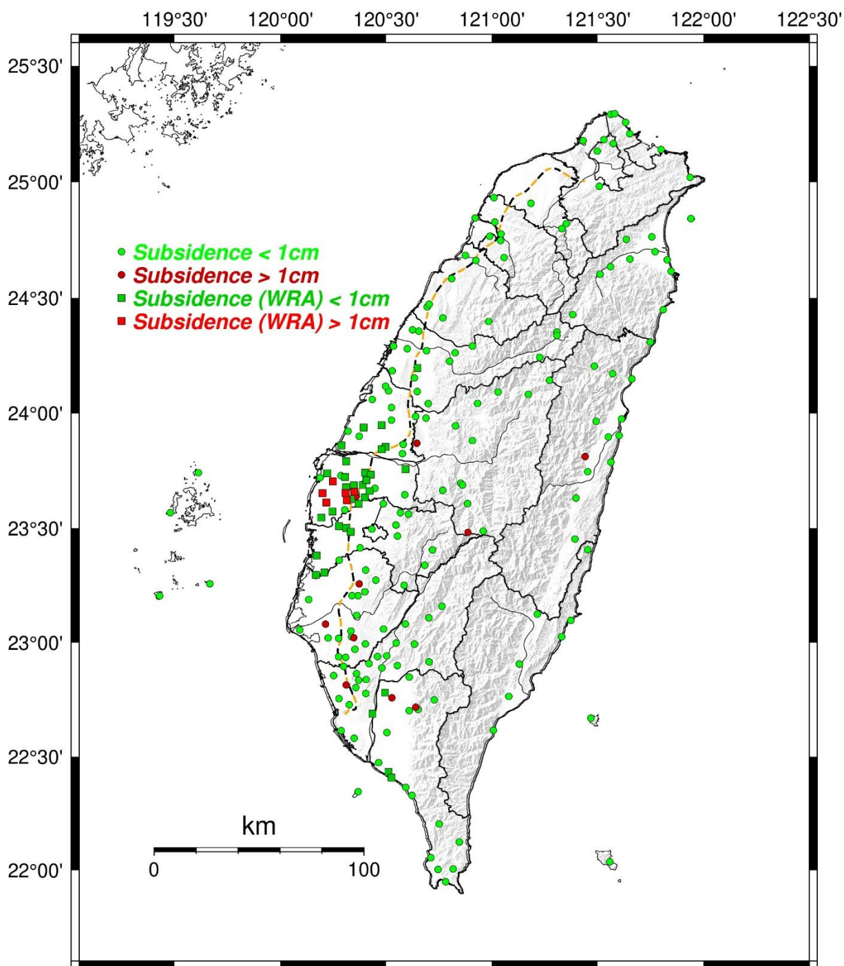
圖 1 114 年 10 月全臺 GNSS 固定站量測成果分析圖
