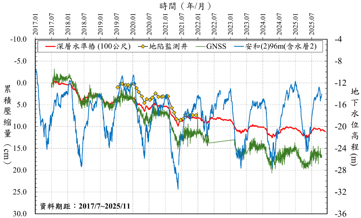
圖 4 嘉義縣灣內國小 106/7~114/10 監測成果分析圖
