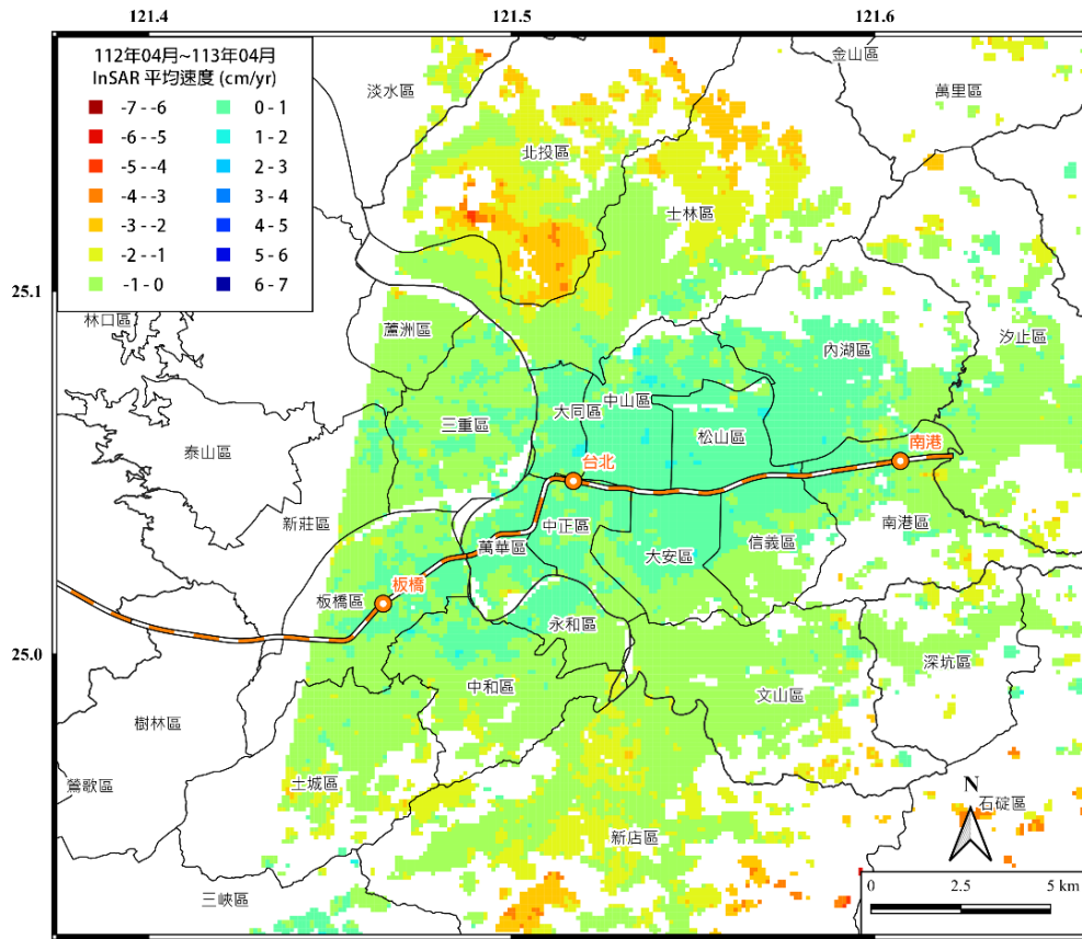
圖 5 臺北地區 112 年 04 月~113 年 04 月之平均位移速度場
