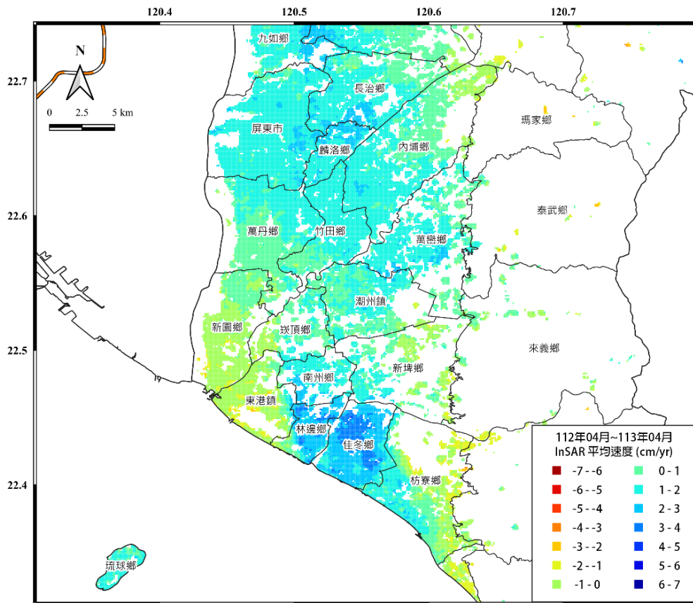
圖 7 屏東地區 112 年 04 月~113 年 04 月之平均位移速度場
