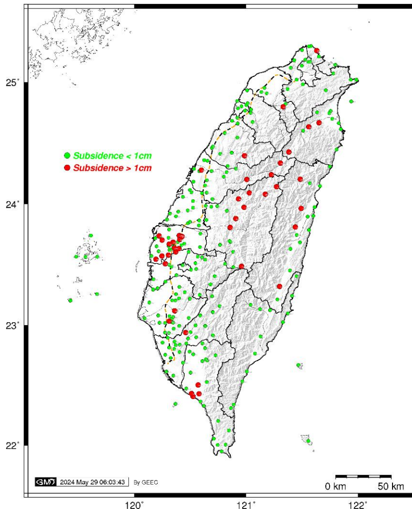
圖 1 113 年 4 月全臺 GNSS 固定站量測成果分析圖
