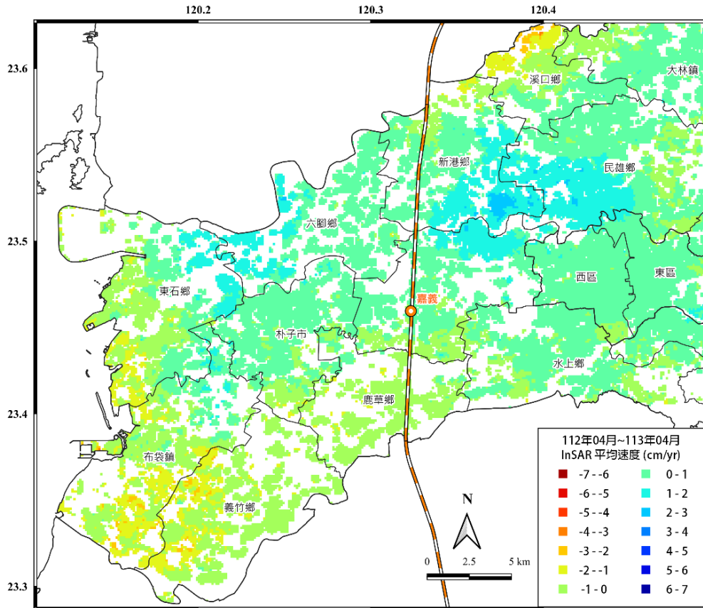
圖 6 嘉義地區 112 年 04 月~113 年 04 月之平均位移速度場
