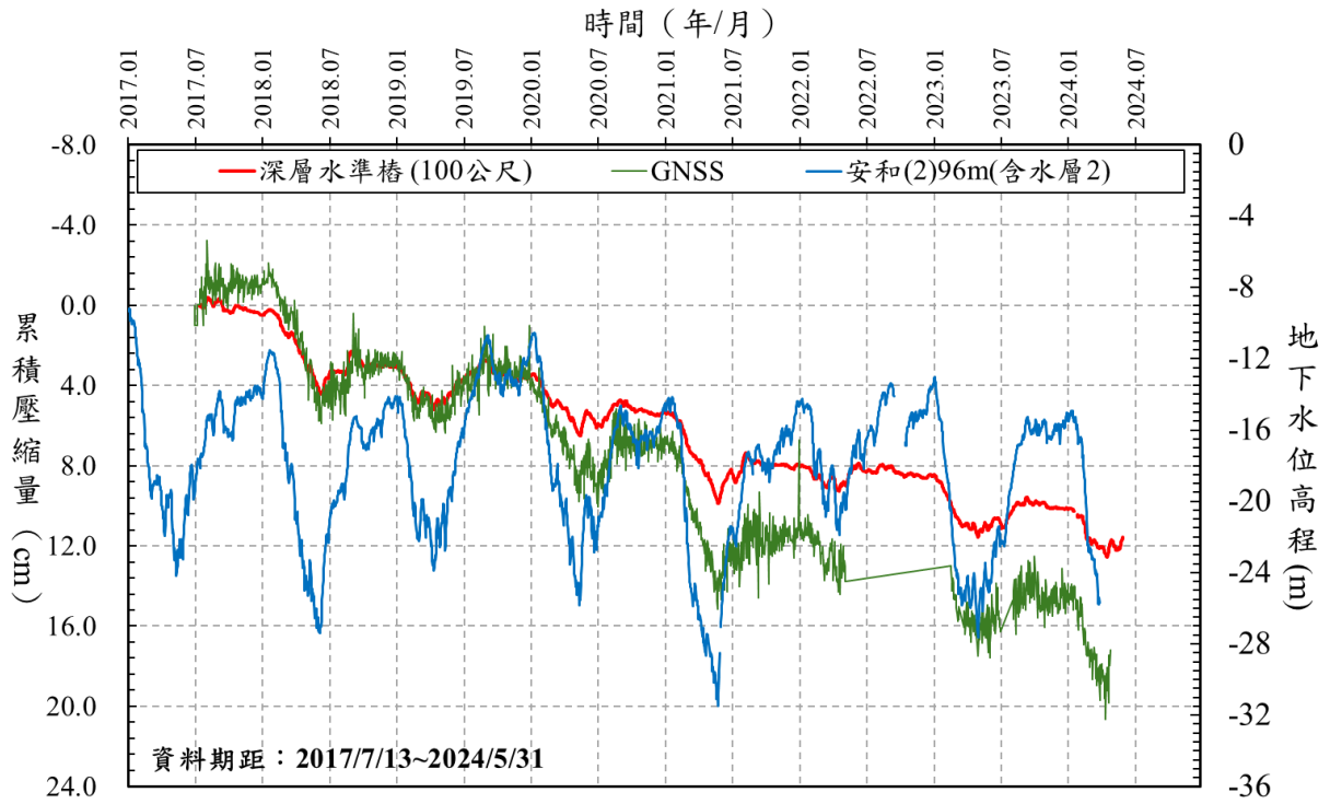
圖 4 嘉義縣灣內國小 106/7~113/5 監測成果分析圖
