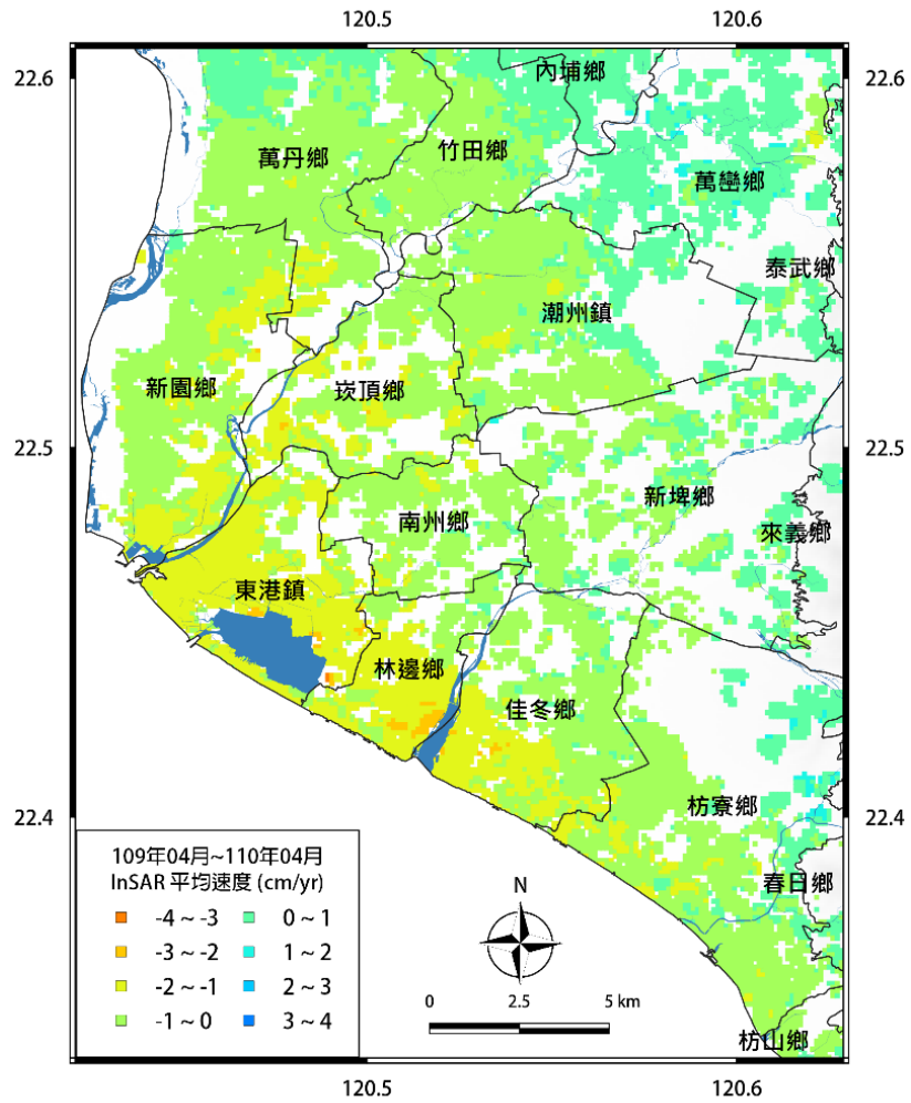
圖 22 屏東地區 109 年 4 月~110 年 4 月之平均位移速度場
