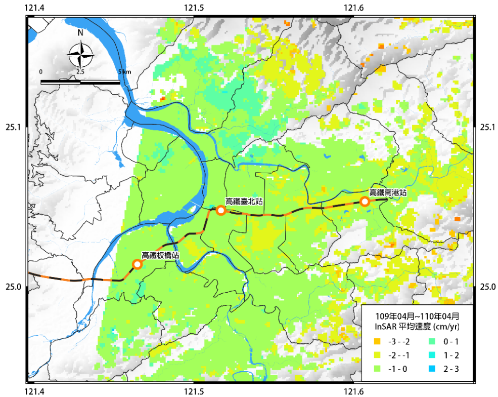
圖 20 臺北地區 109 年 4 月~110 年 4 月之平均位移速度場
