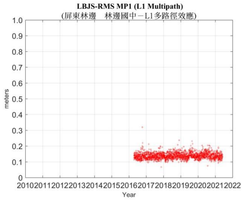
林邊國中 GNSS 固定站訊號品質分析圖
