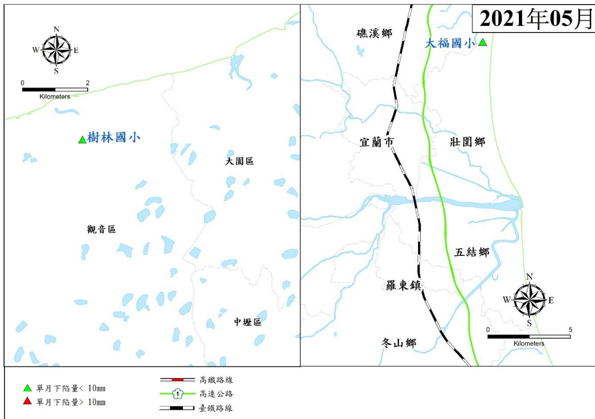
圖 7 宜蘭與桃園地區 110 年 5 月(單月)地陷監測井量測成果圖
