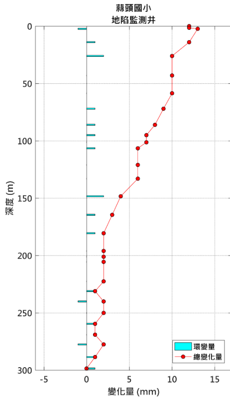
圖 13 蒜頭國小潭墘分校地陷監測井 2 月環變量分析圖
