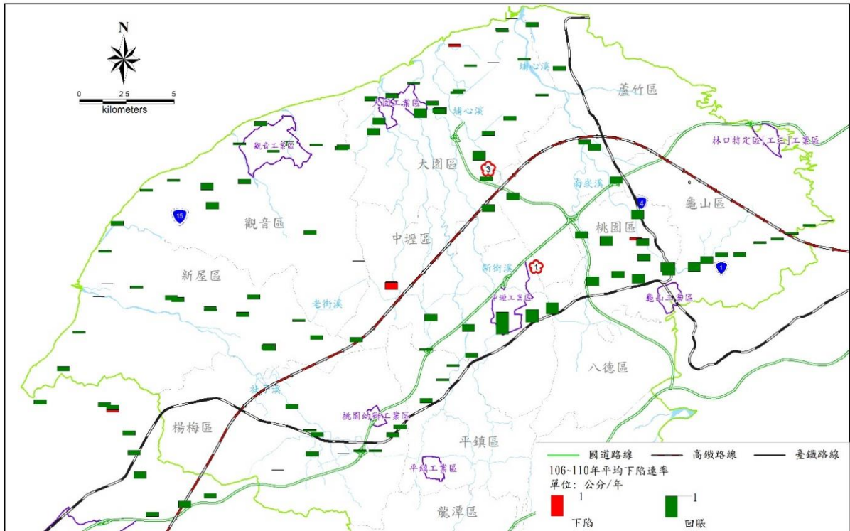
圖 1 桃園地區 106~110 年水準檢測成果圖
