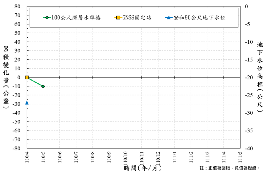
圖 19 嘉義縣灣內國小 110/4~110/5 監測成果比較圖
