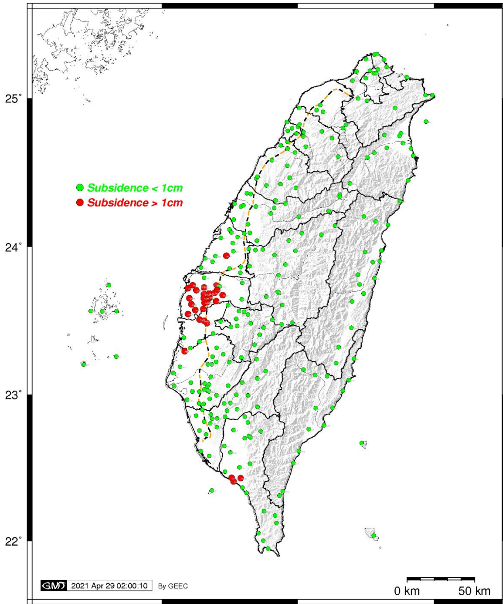
圖 15 110 年 4 月全臺 GNSS 固定站量測成果分析圖
