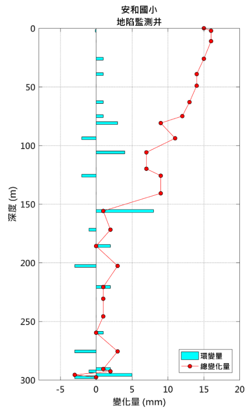
圖 10 高雄與屏東地區 110 年 5 月(單月)地陷監測井量測成果圖
