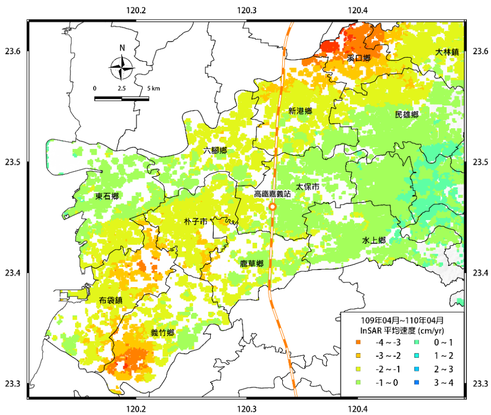
圖 21 嘉義地區 109 年 4 月~110 年 4 月之平均位移速度場
