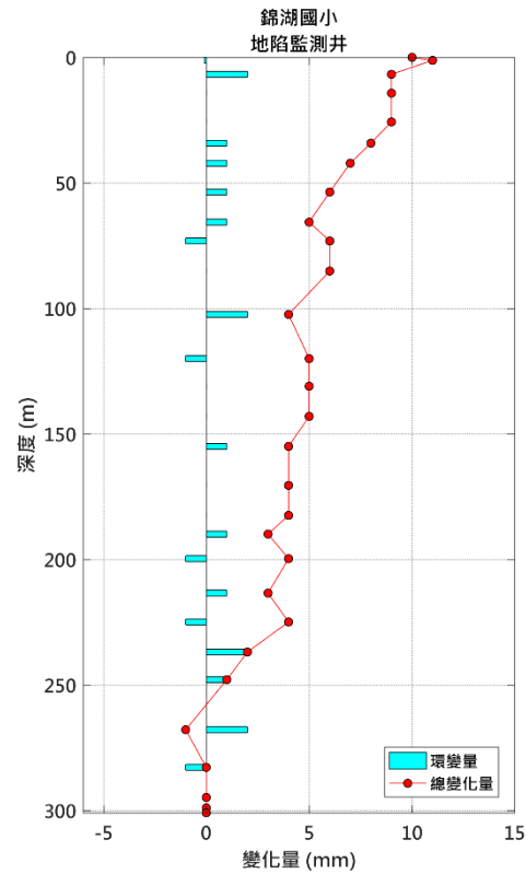
圖 14 錦湖國小地陷監測井 2 月環變量分析圖
