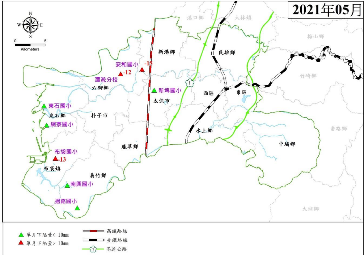
圖 8 嘉義地區 110 年 5 月(單月)地陷監測井量測成果圖
