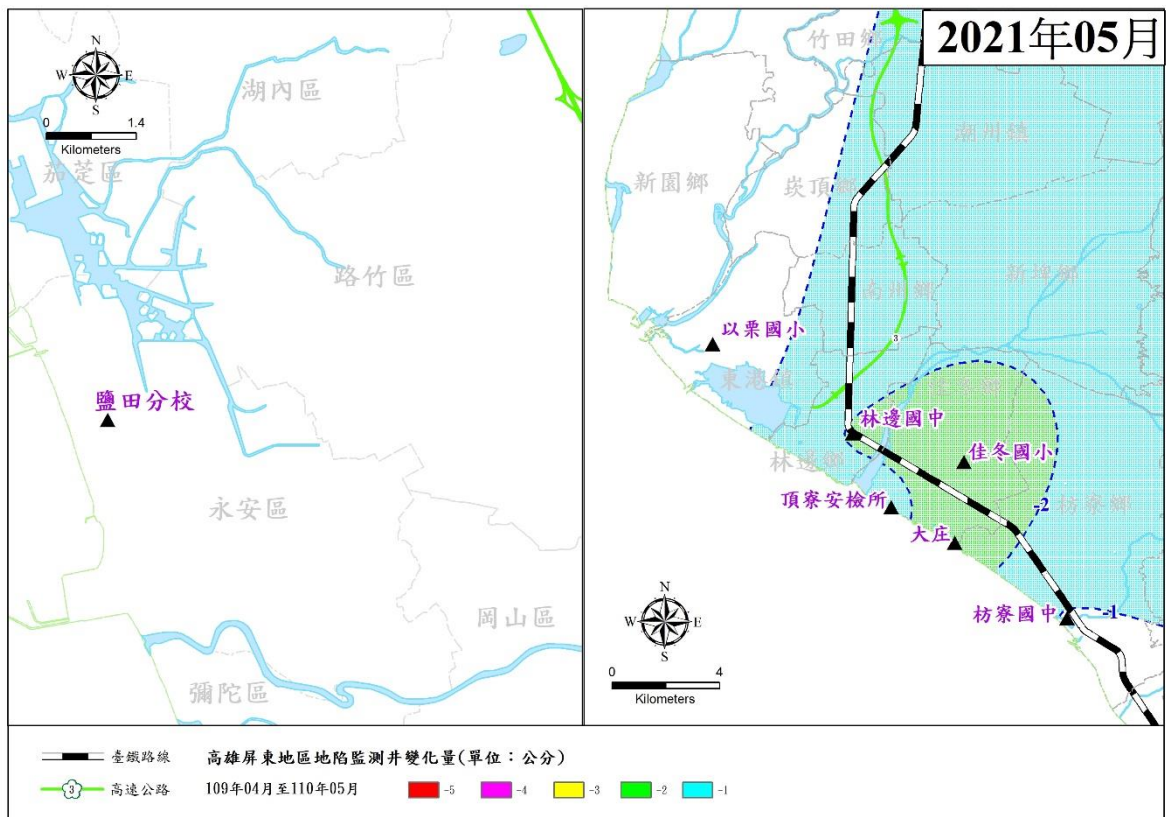
圖 5 高雄與屏東地區 109 年 4 月~110 年 5 月地陷監測井累積變化量圖
