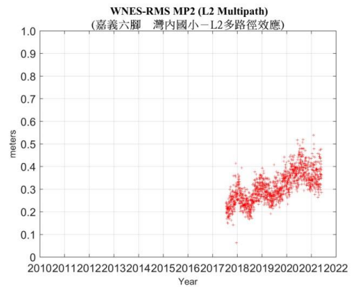
灣內國小 GNSS 固定站訊號品質分析圖
