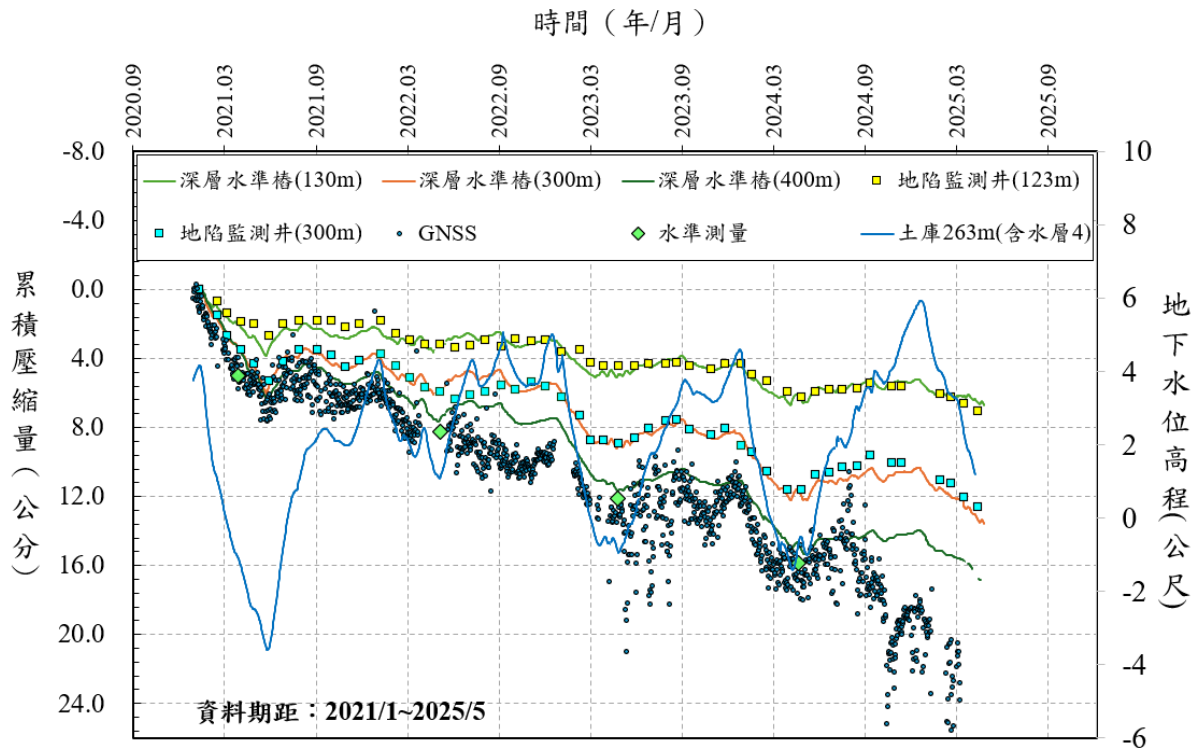
圖 6 雲林縣土庫國中 103/12~114/5 監測成果比較圖
