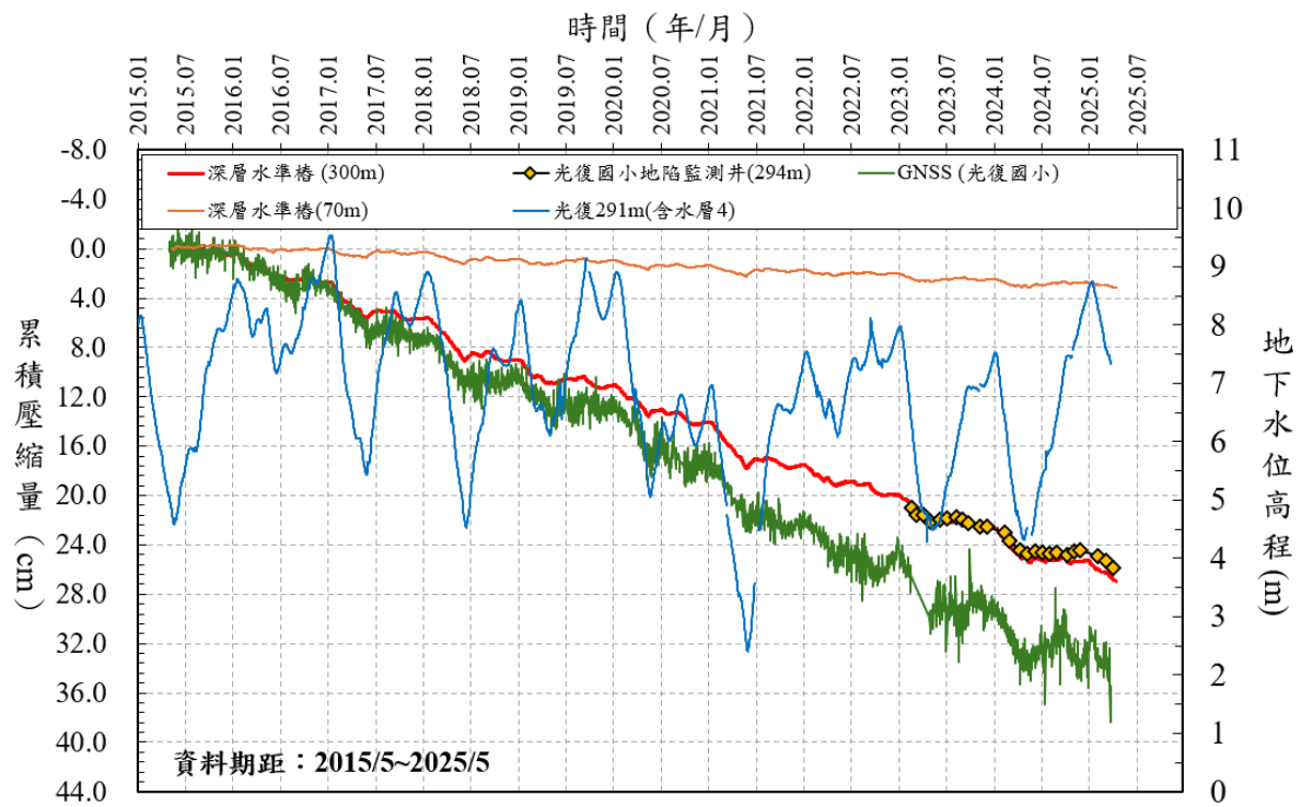
圖 8 雲林縣中科虎尾園區 104/11~114/5 監測成果比較圖
