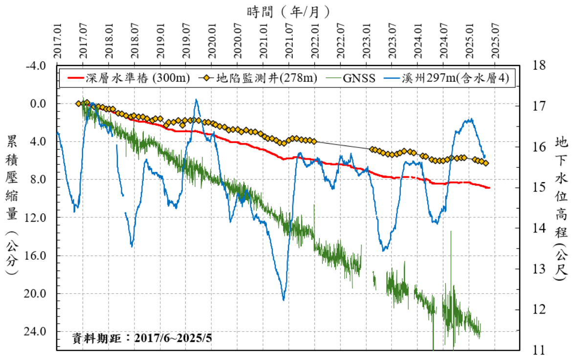
圖 5 彰化縣溪州國小 106/6~114/5 監測成果比較圖
