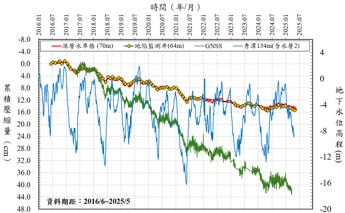
圖 7 雲林縣秀潭國小 105/6~114/5 監測成果比較圖
