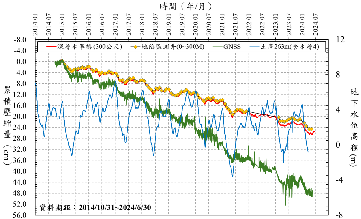
圖 6 雲林縣土庫國中 103/12~113/6 監測成果比較圖
