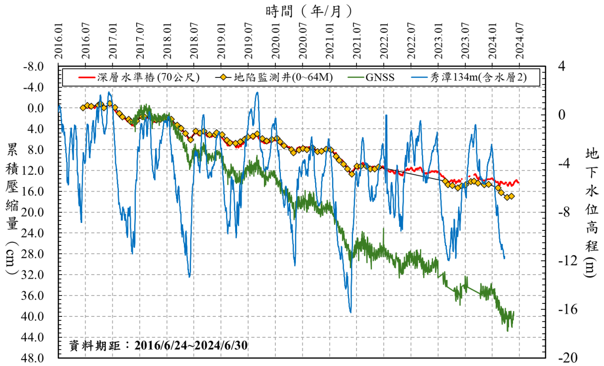
圖 7 雲林縣秀潭國小 105/6~113/6 監測成果比較圖
