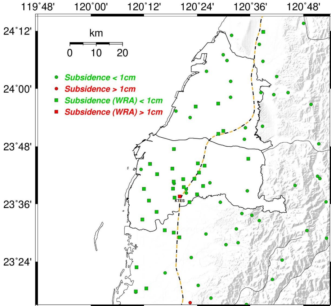
圖 3 113 年 5 月彰雲地區 GNSS 固定站量測成果分析圖
