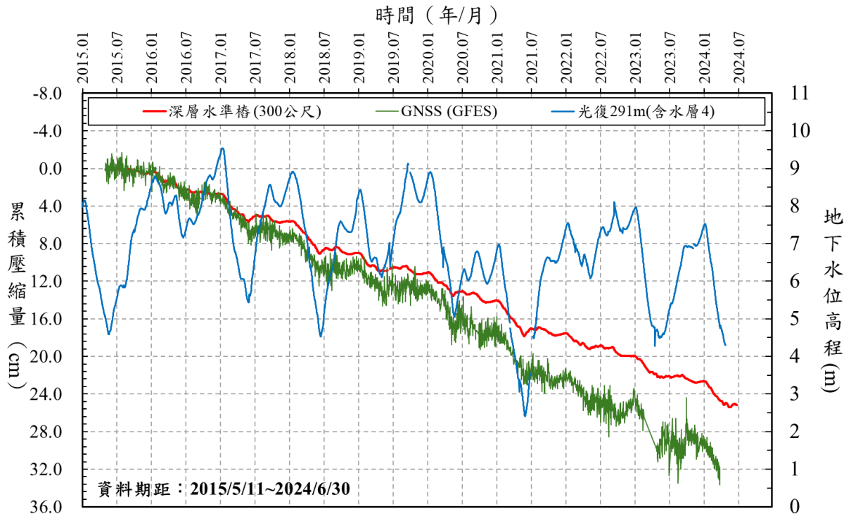
圖 8 雲林縣中科虎尾園區 104/11~113/6 監測成果比較圖
