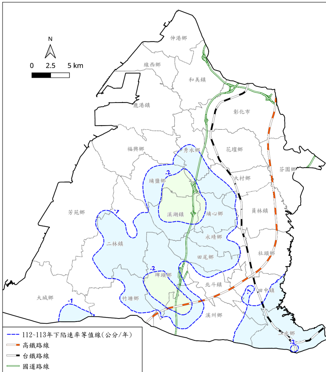
圖 1 113 年彰化地區下陷速率等值線圖
