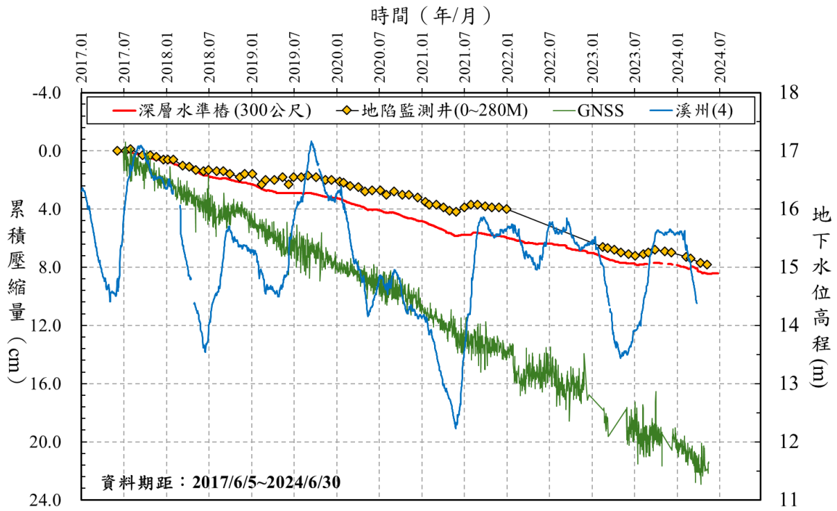
圖 5 彰化縣溪州國小 106/7~113/6 監測成果比較圖
