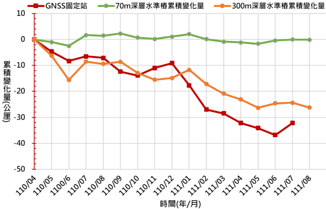
圖 5 雲林縣中科虎尾園區 110/4~111/7 監測成果比較圖
