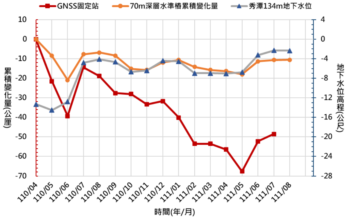
圖 4 雲林縣秀潭國小 110/4~111/8 監測成果比較圖
