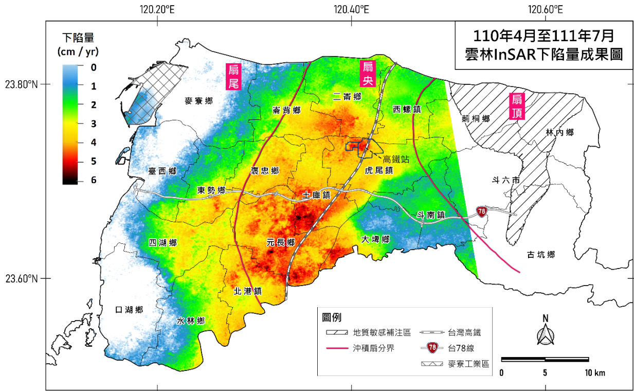
圖 7 110 年 4 月至 111 年 7 月雲林地區 InSAR 下陷成果圖 註：正值代表下陷，負值代表回脹
