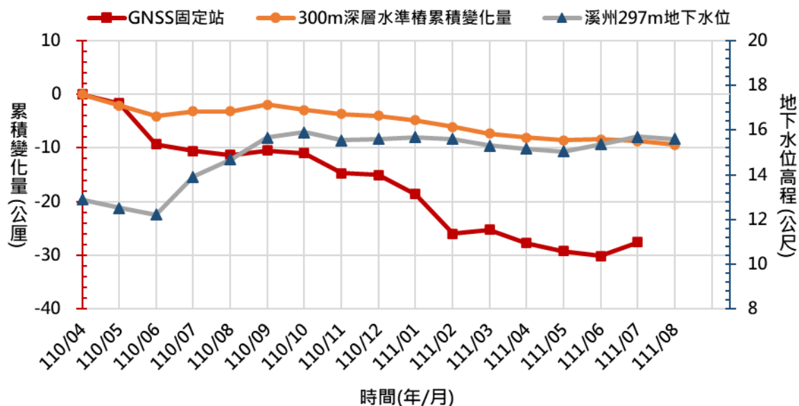
圖 2 彰化縣溪州國小 110/4~111/8 監測成果比較圖
