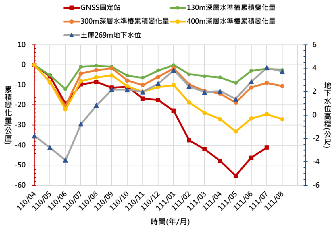
圖 3 雲林縣土庫國中 110/4~111/8 監測成果比較圖
