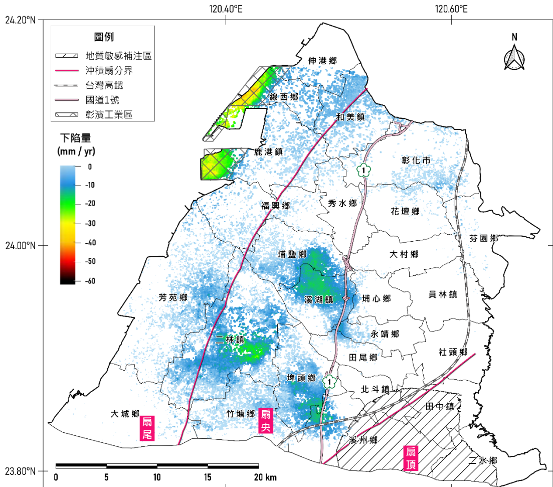
圖5 110年4月至111年3月彰化地區 InSAR 下陷成果圖
