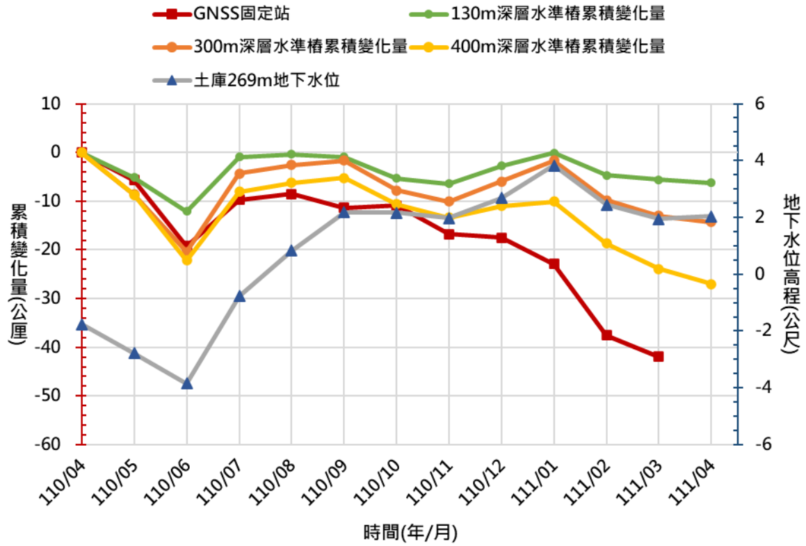
圖 2 雲林縣土庫國中 110/4~111/4 監測成果比較圖
