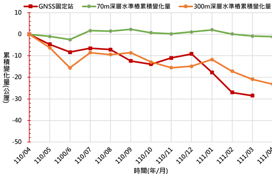
圖 4 雲林縣中科虎尾園區 110/4~111/4 監測成果比較圖
