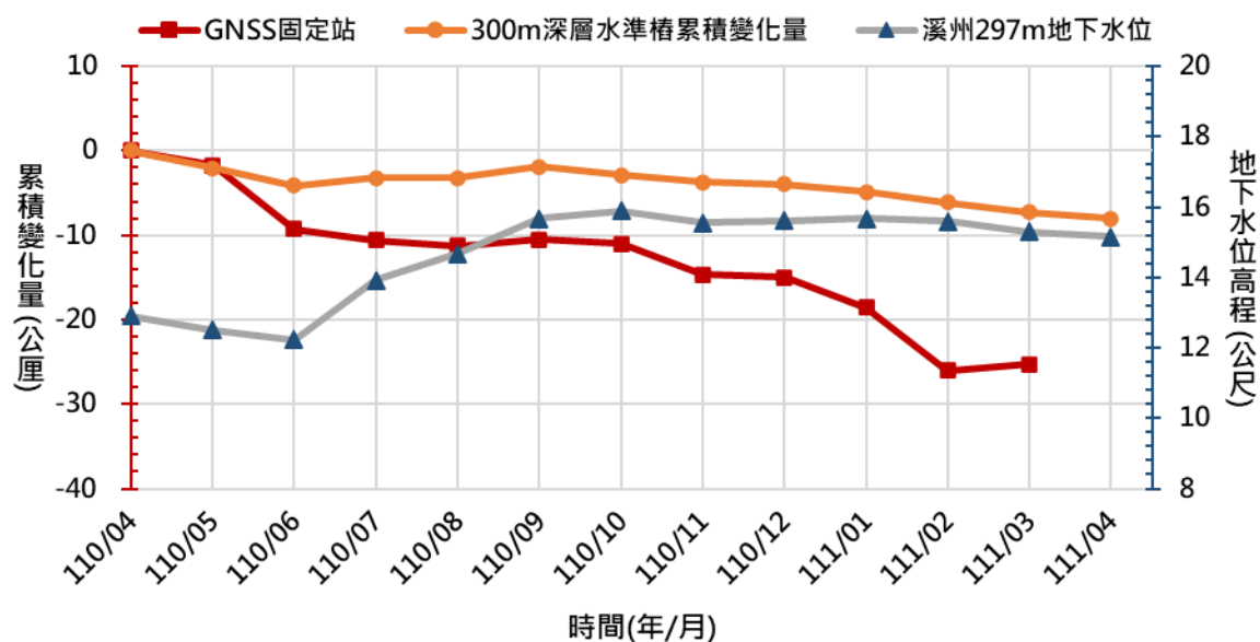
圖 1 彰化縣溪州國小 110/4~111/4 監測成果比較圖
