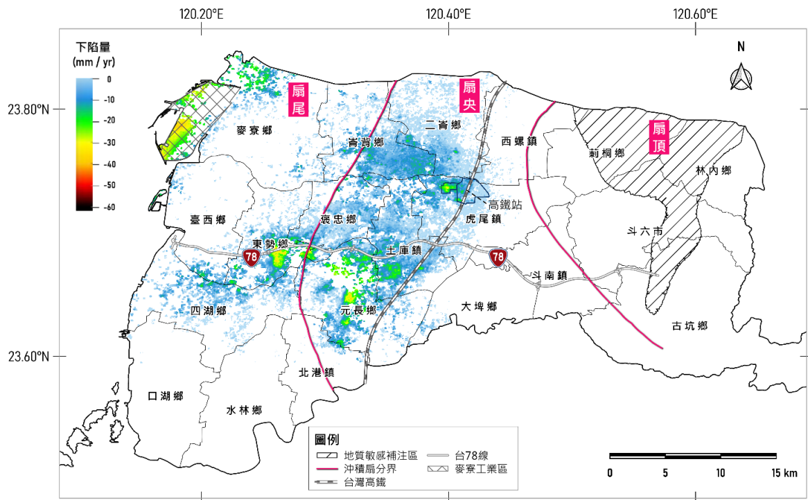
圖 6 110 年 4 月至 111 年 3 月雲林地區 InSAR 下陷成果圖
