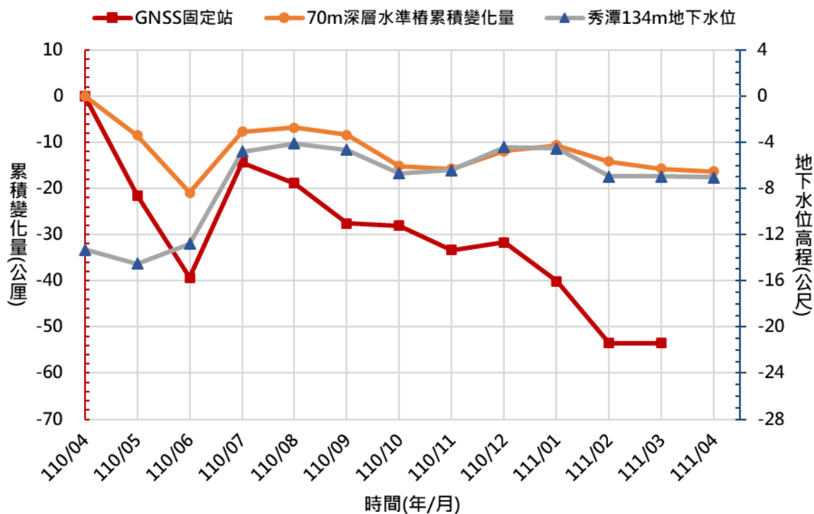
圖 3 雲林縣秀潭國小 110/4~111/4 監測成果比較圖
