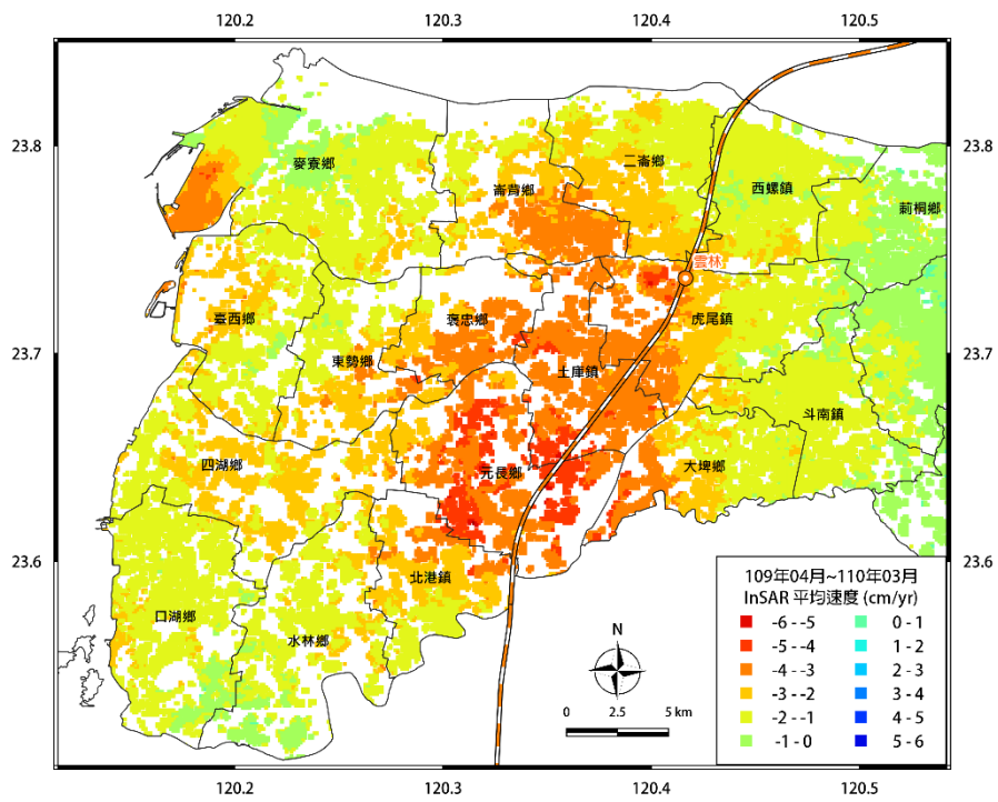
圖 25 雲林地區 109 年 4 月~110 年 3 月之平均位移速度場
