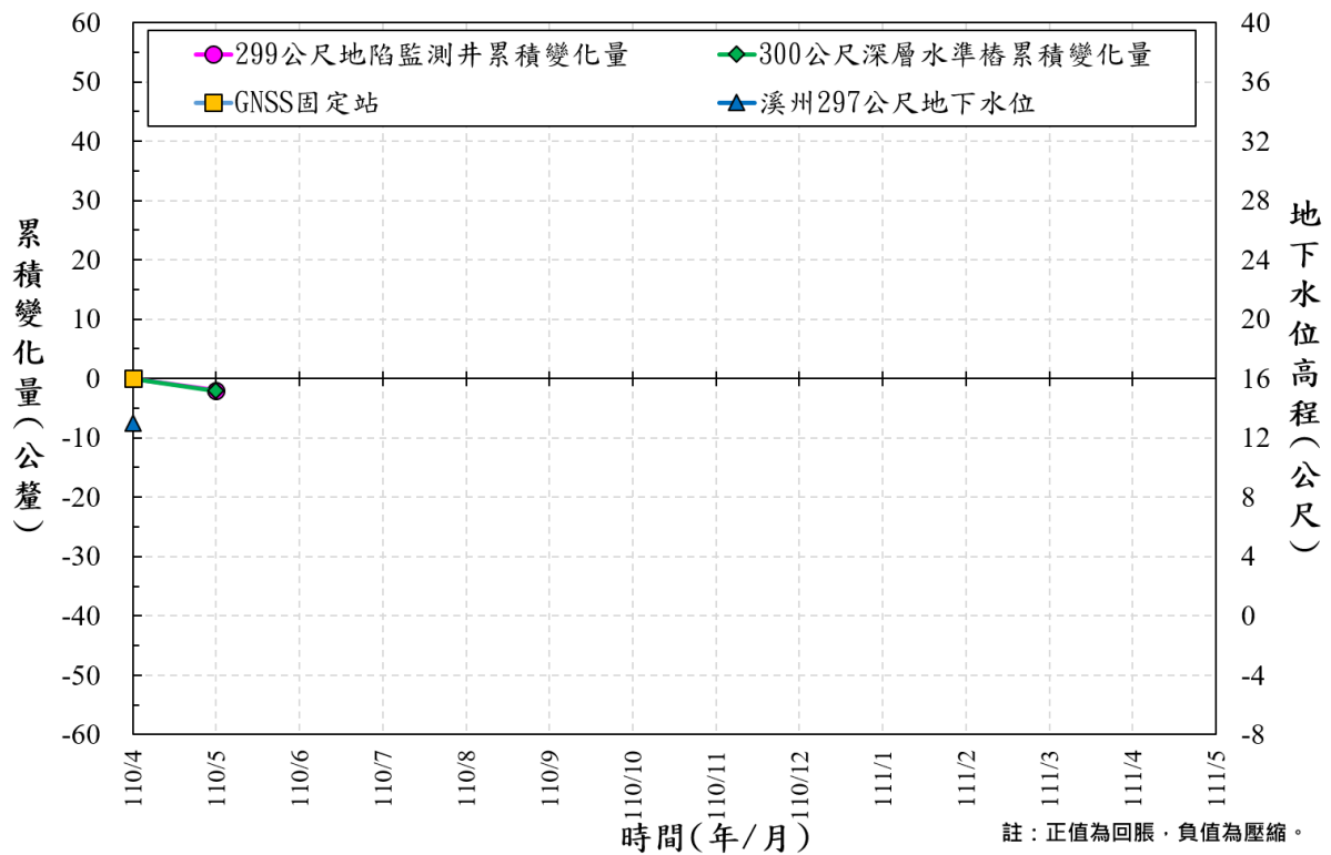
圖 19 彰化縣溪州國小 110/4~110/5 監測成果比較圖
