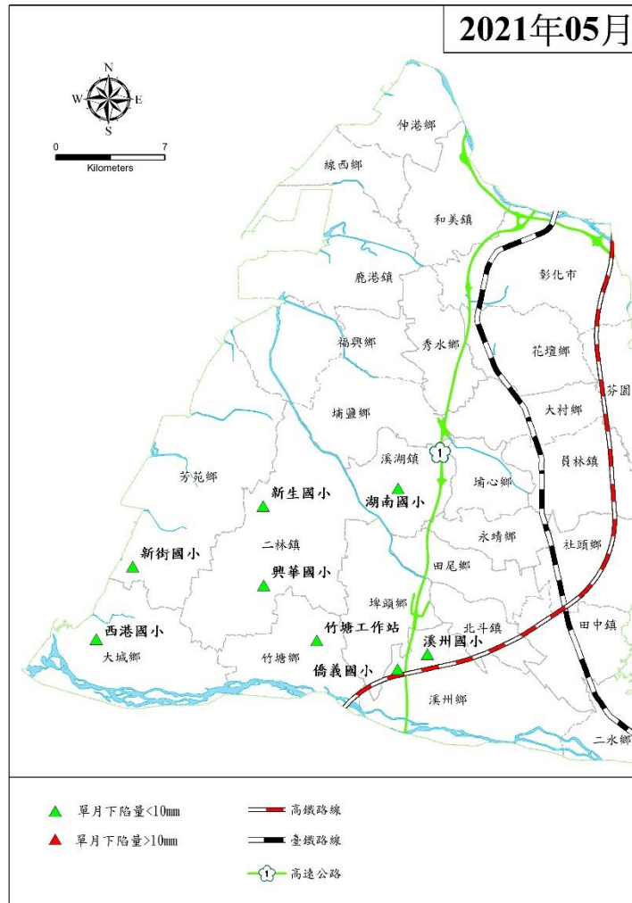
圖 6 彰化地區 110 年 5 月(單月)地陷監測井量測成果圖
