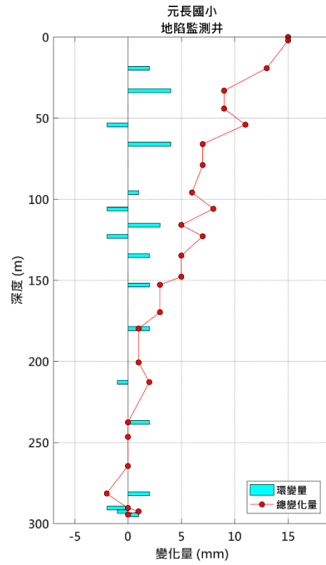
圖 13 元長國小地陷監測井 5 月環變量分析圖
