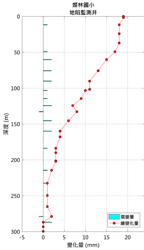
圖 12 水燦林國小地陷監測井 5 月環變量分析圖
