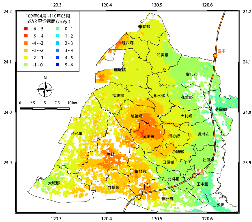
圖 23 彰化地區 109 年 4 月~110 年 3 月之平均位移速度場
