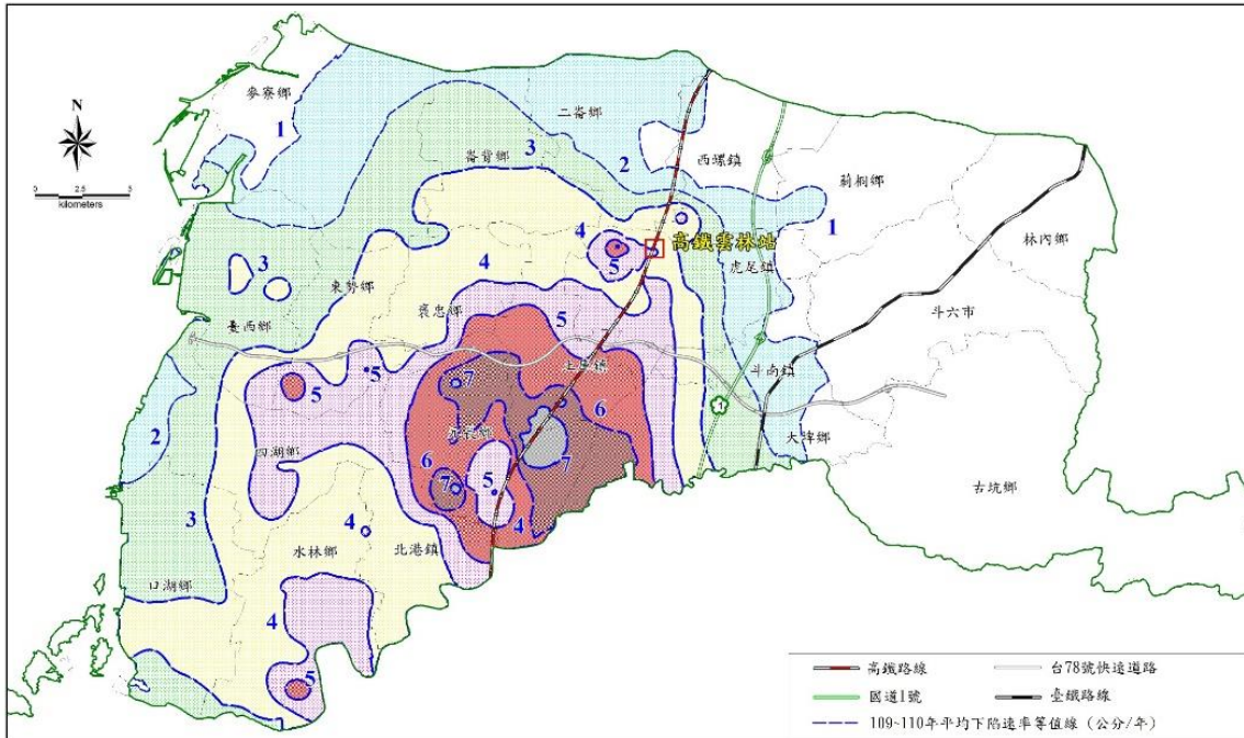
圖 1 雲林地區 110 年下陷速率等值線圖
