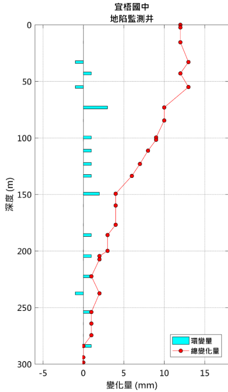
圖 18 宜梧國中地陷監測井 5 月環 變量分析圖
