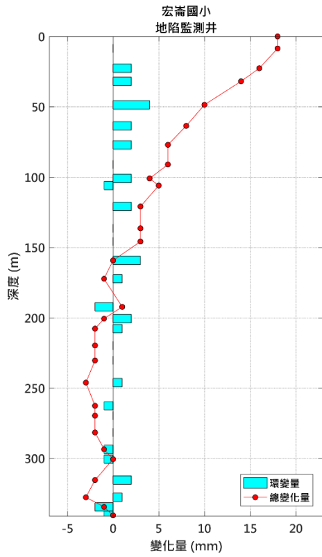
圖 16 宏崙國小地陷監測井 5 月環 變量分析圖
