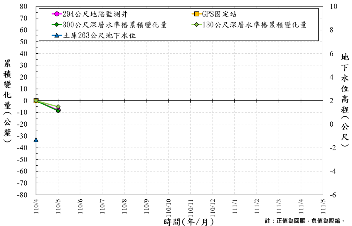
圖 20 雲林縣土庫國中 110/4~110/5 監測成果比較圖
