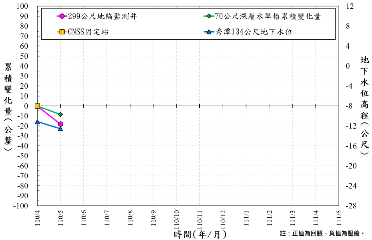
圖 21 雲林縣秀潭國小 110/4~110/5 監測成果比較圖
