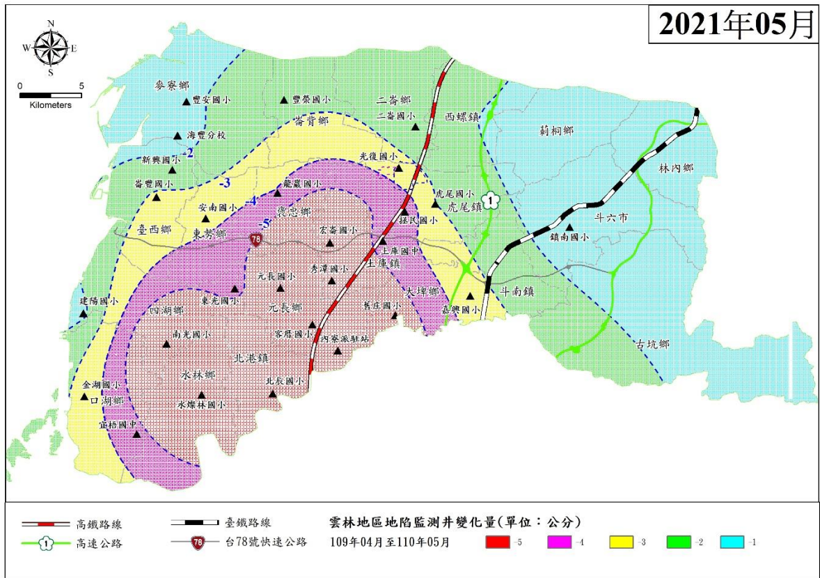
圖 4 雲林地區 109 年 4 月~110 年 5 月地陷監測井累積變化量圖 註：正值為回脹，負值為下陷。
