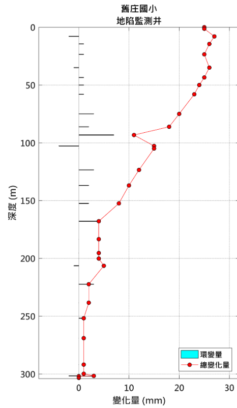
0.2 圖 15 舊庄國小地陷監測井 5 月環變量分析圖
