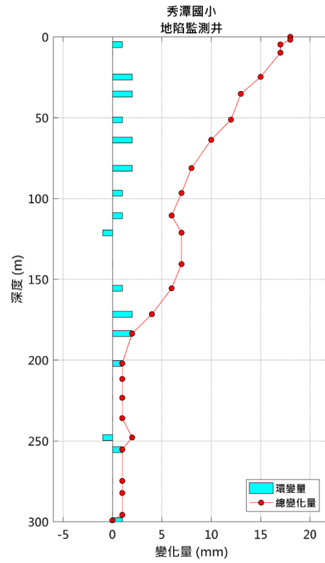
圖 17 秀潭國小地陷監測井 5 月環 變量分析圖
