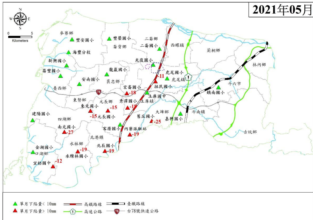
圖 7 雲林地區 110 年 5 月(單月)地陷監測井量測成果圖
