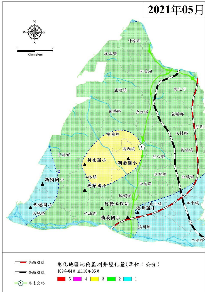
圖3 彰化地區 109 年 4 月~110 年 5 月地陷監測井累積變化量圖 註：正值為回脹，負值為下陷。
