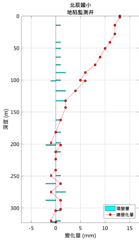
圖 10 北辰國小地陷監測井 3 月環變量分析圖
