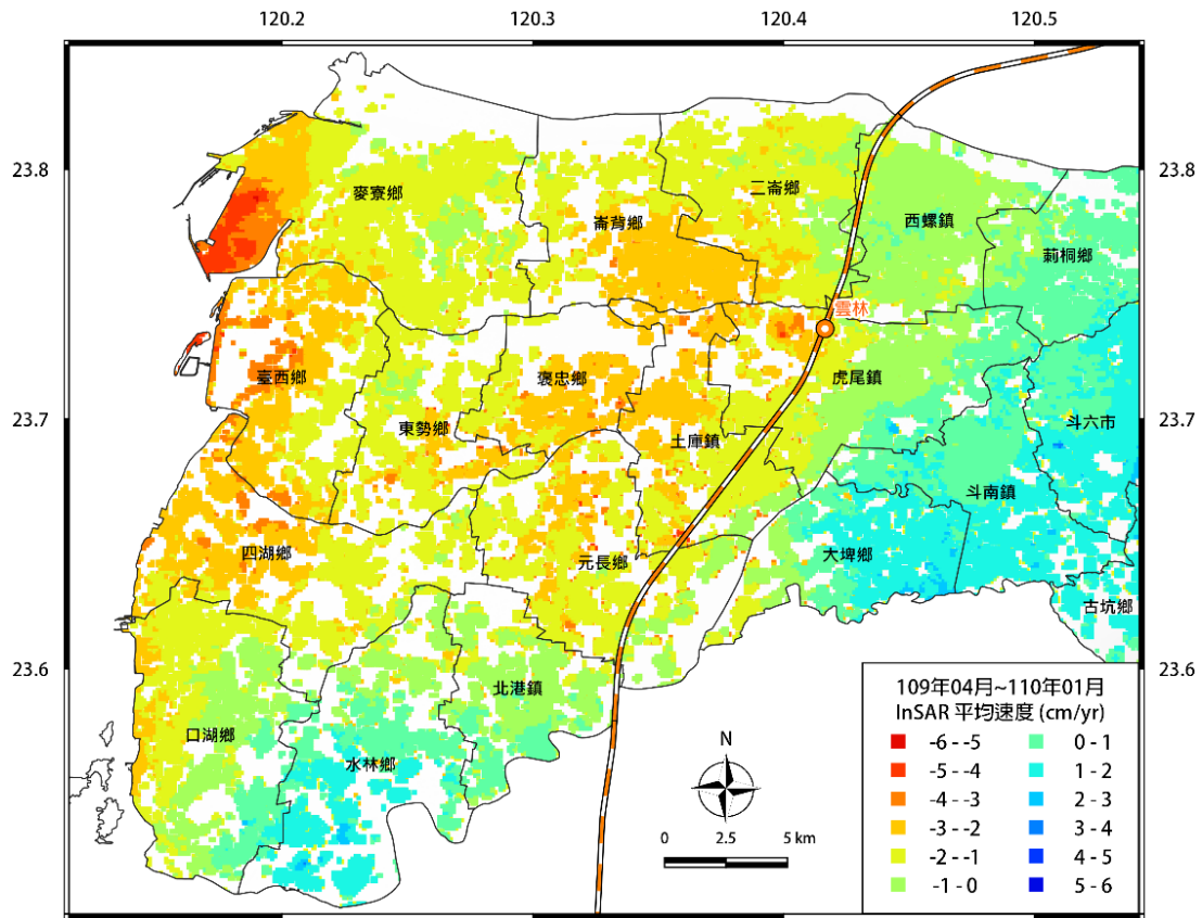
圖 22 雲林地區 109 年 4 月~110 年 1 月之平均位移速度場
