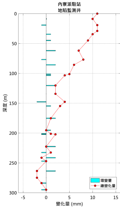
圖 8 內寮派駐站地陷監測井 3 月環變量分析圖
