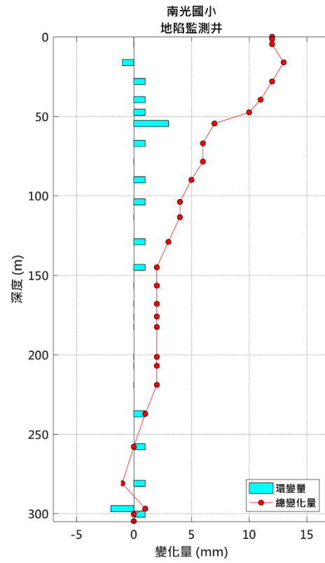
圖 13 南光國小地陷監測井 3 月環變量分析圖
