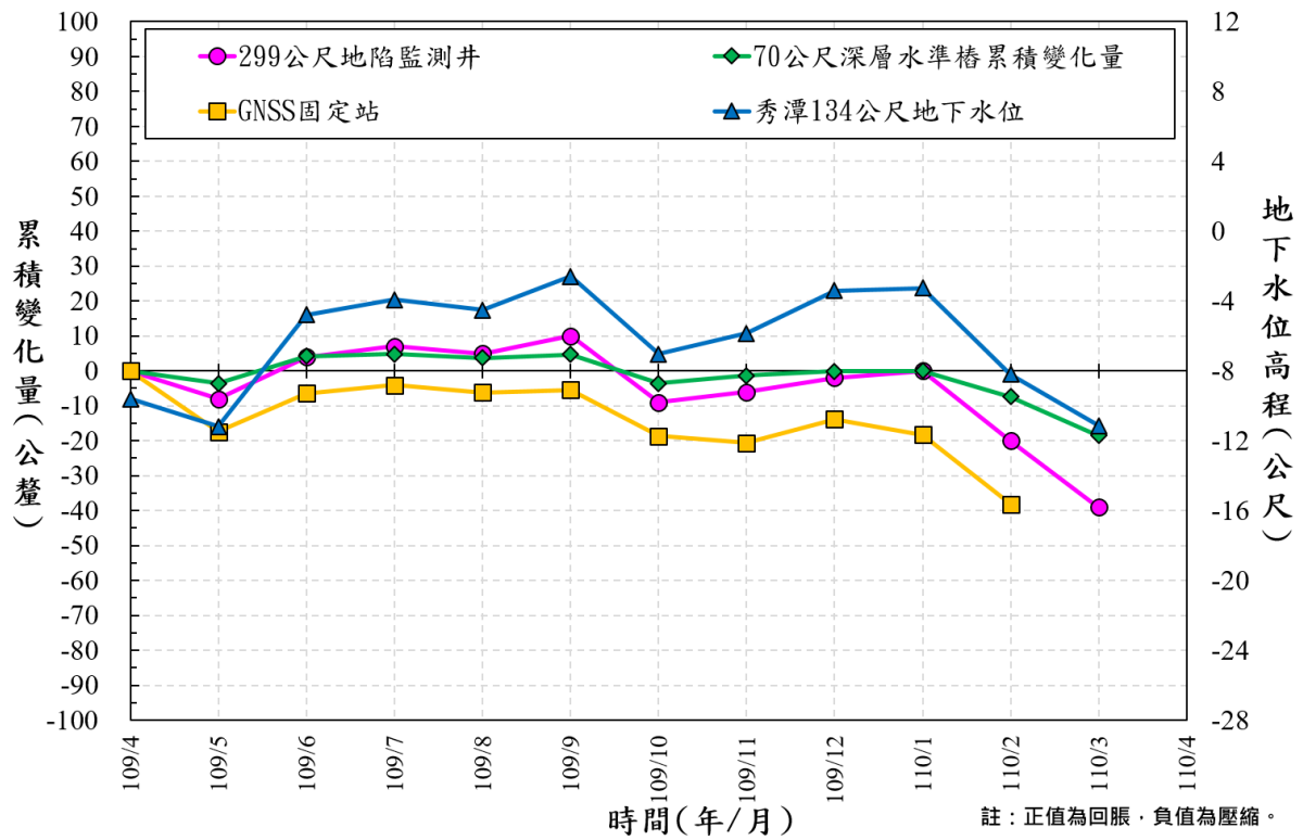
圖 18 雲林縣秀潭國小 109/4~110/3 監測成果比較圖
