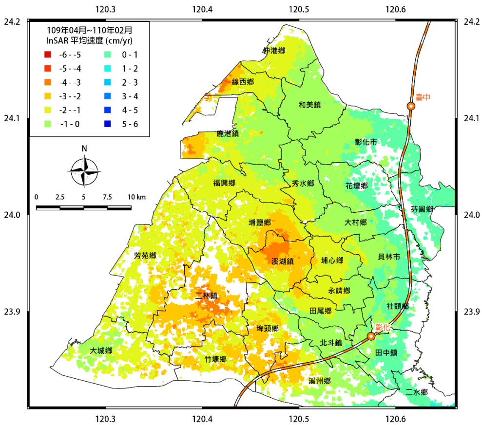
圖 21 彰化地區 109 年 4 月~110 年 2 月之平均位移速度場
