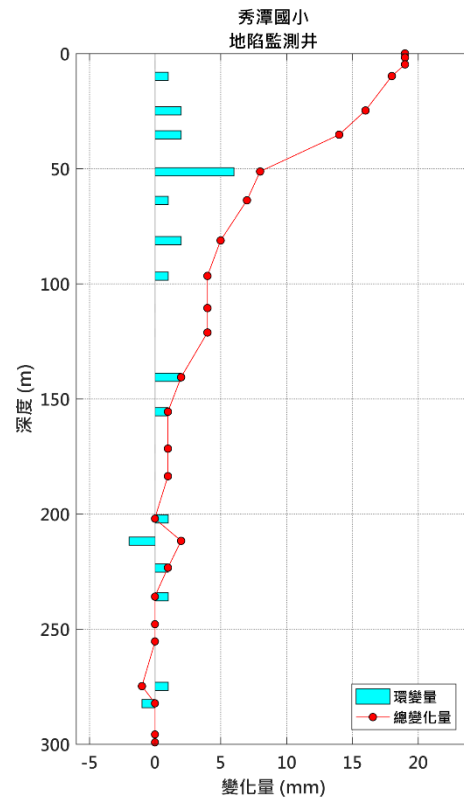
圖 11 秀潭國小地陷監測井 3 月環變量分析圖
