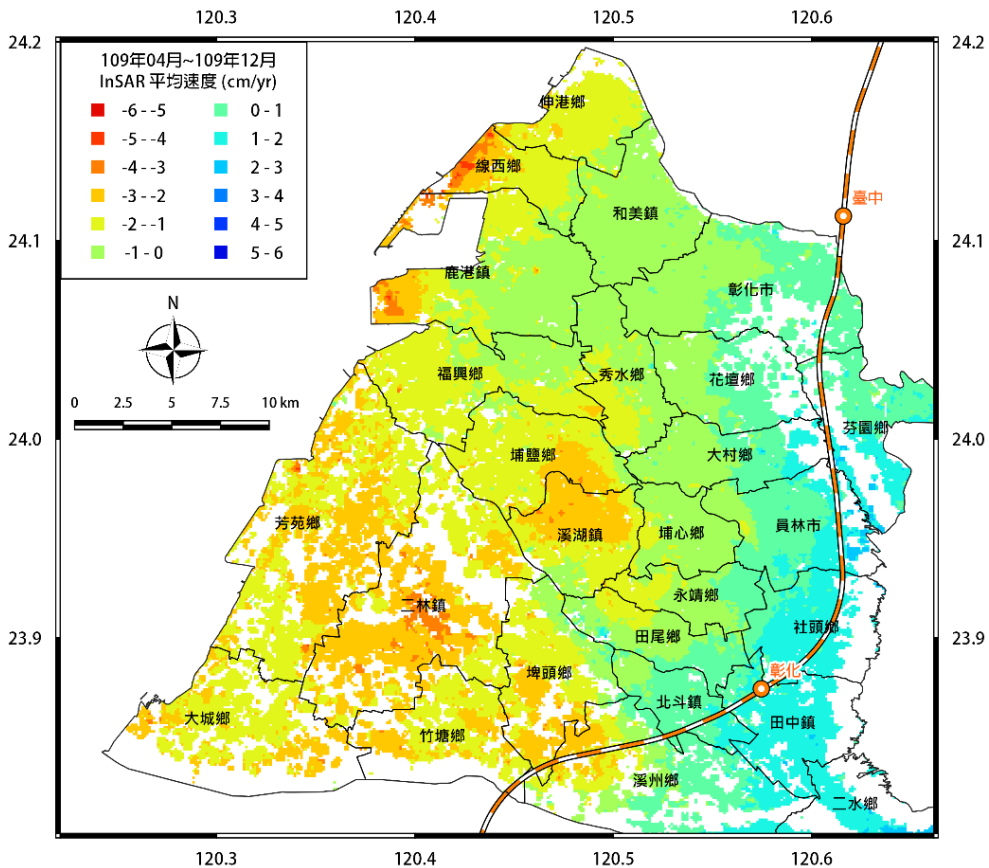
圖 20 彰化地區 109 年 4 月~110 年 1 月之平均位移速度場
