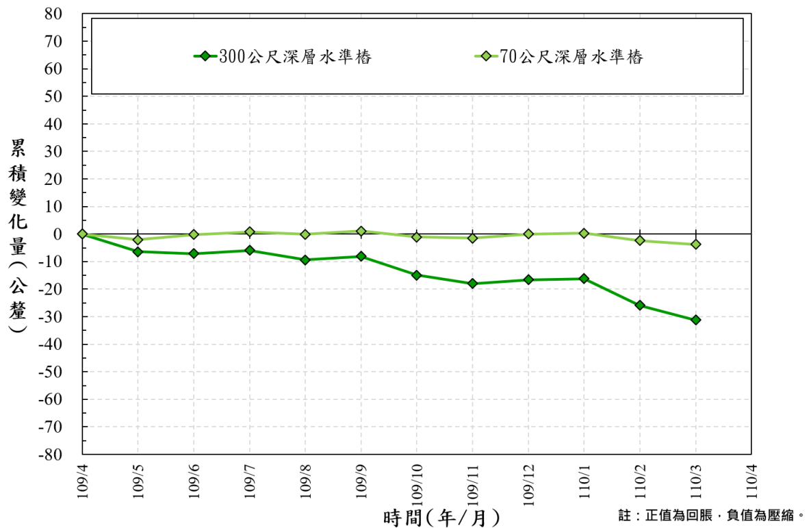
圖 19 雲林縣中科虎尾園區 109/4~110/3 監測成果比較圖
