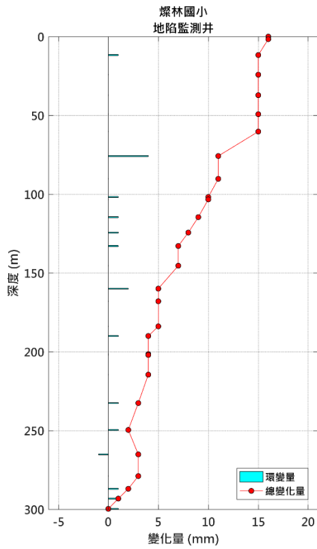
圖 14 水燦林國小地陷監測井 3 月環變量分析圖
