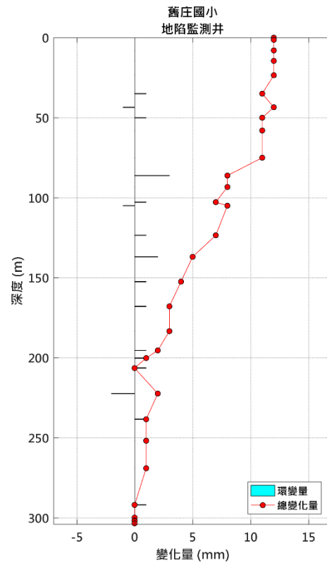
圖 15 舊庄國小地陷監測井 3 月環變量分析圖
