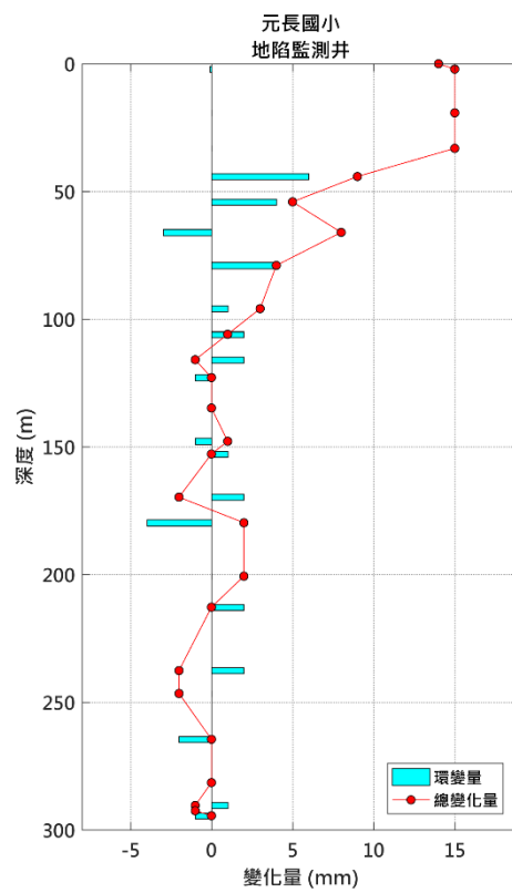
圖 7 元長國小地陷監測井 3 月環變量分析圖
