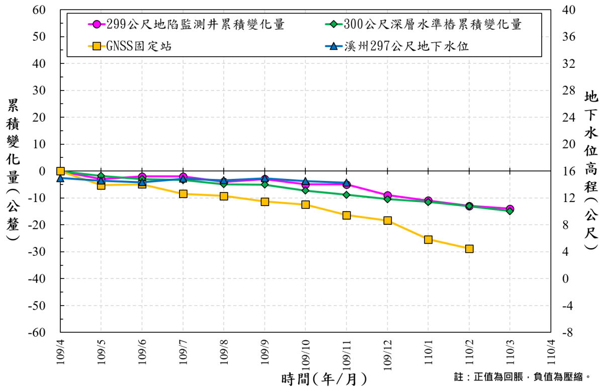
圖 16 彰化縣溪州國小 109/4~110/3 監測成果比較圖
