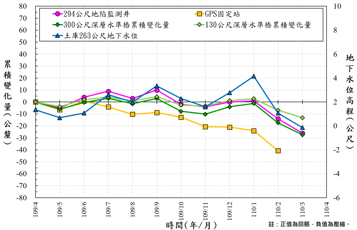
圖 17 雲林縣土庫國中 109/4~110/3 監測成果比較圖
