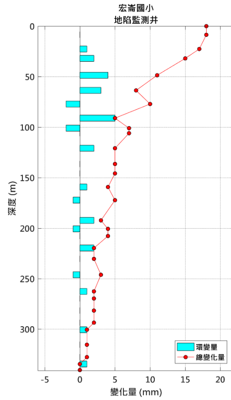
圖 9 宏崙國小地陷監測井 3 月環變量分析圖
