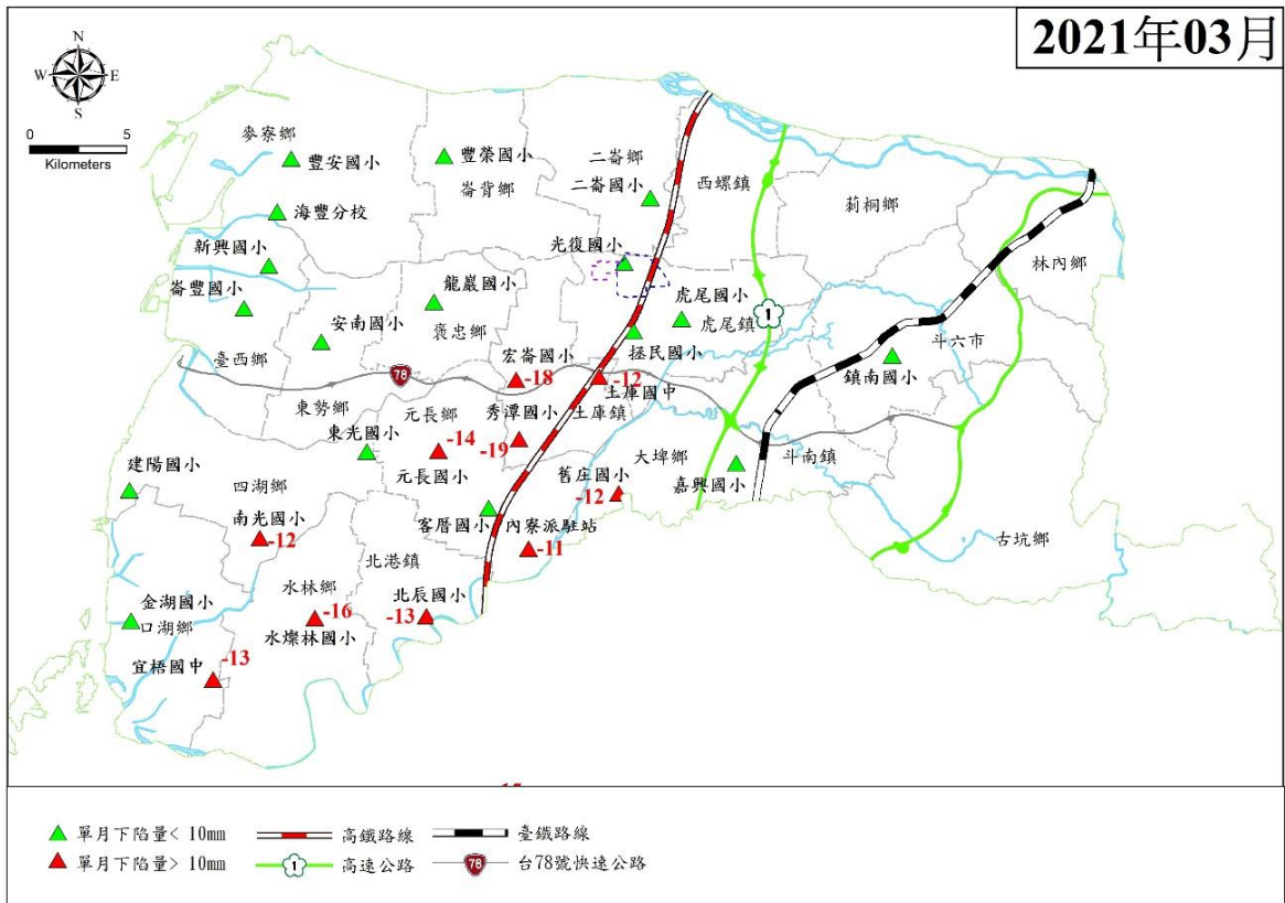
圖 5 雲林地區 110 年 3 月(單月)地陷監測井量測成果圖
