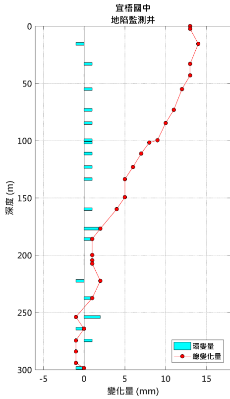
圖 12 宜梧國中地陷監測井 3 月環變量分析圖
