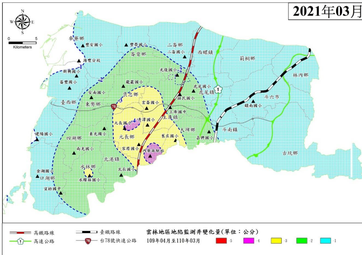
圖 2 雲林地區 109 年 4 月~110 年 3 月地陷監測井累積變化量圖
