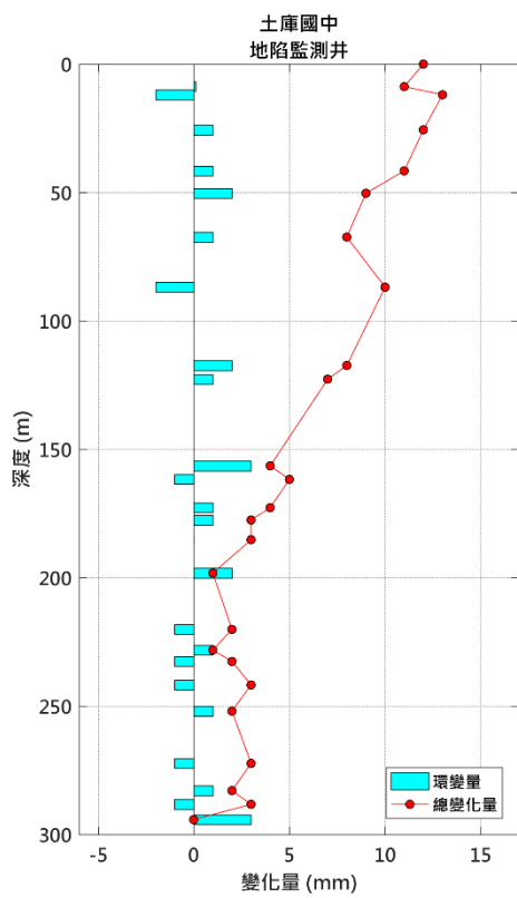
圖 6 土庫國中地陷監測井 3 月環變量分析圖
