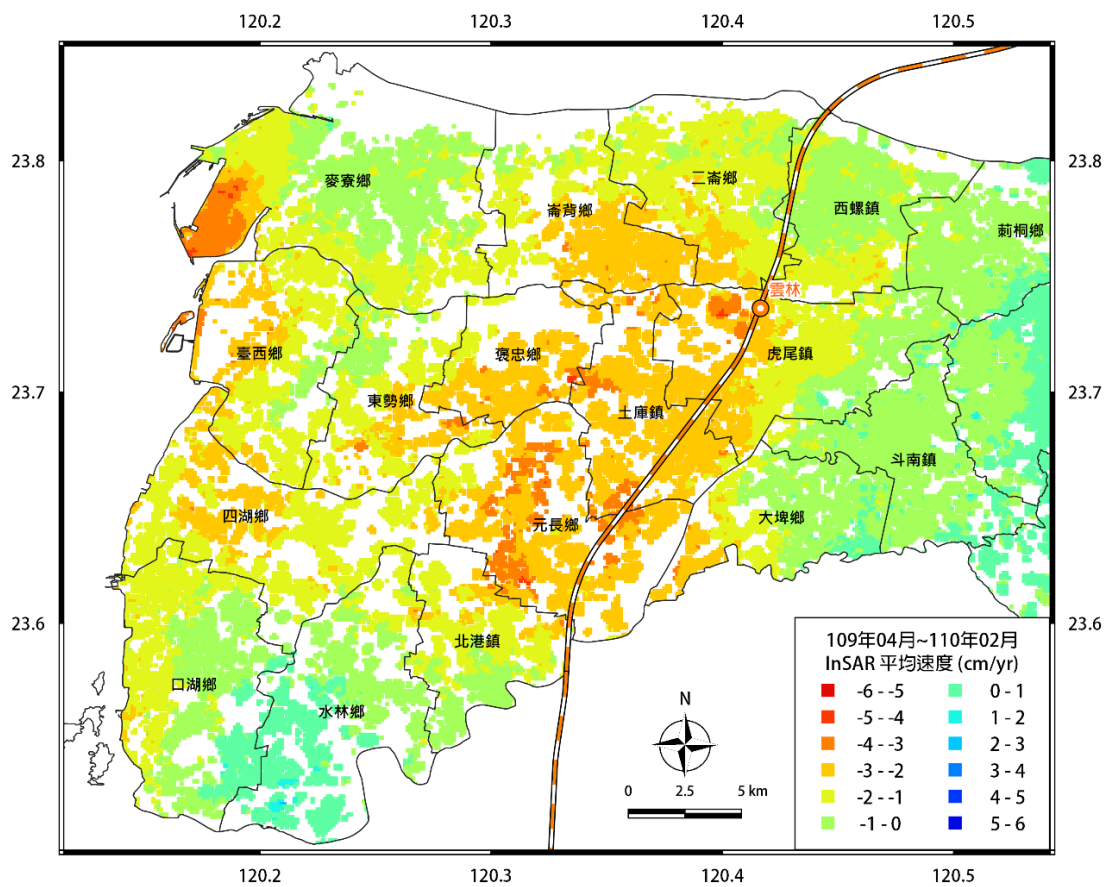
圖 23 雲林地區 109 年 4 月~110 年 2 月之平均位移速度場
