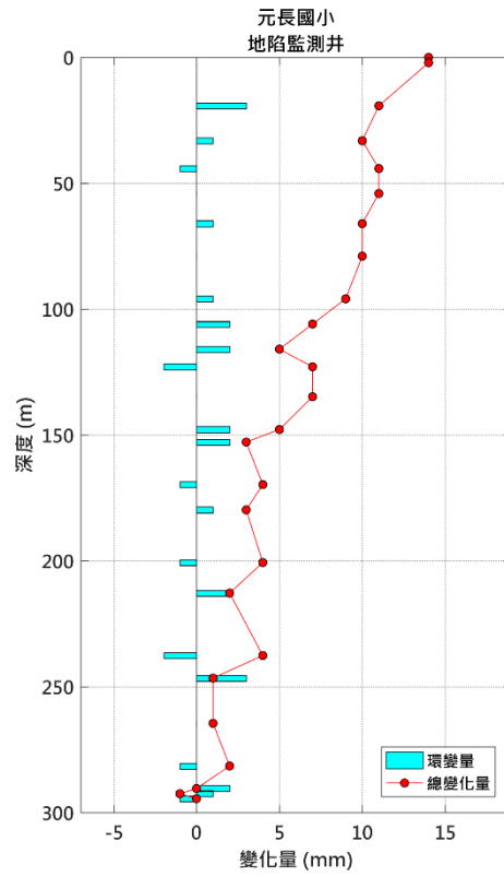
圖 7 元長國小地陷監測井 2 月環變量分析圖
