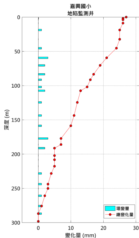
圖 15 嘉興國小地陷監測井 2 月環變量分析圖
