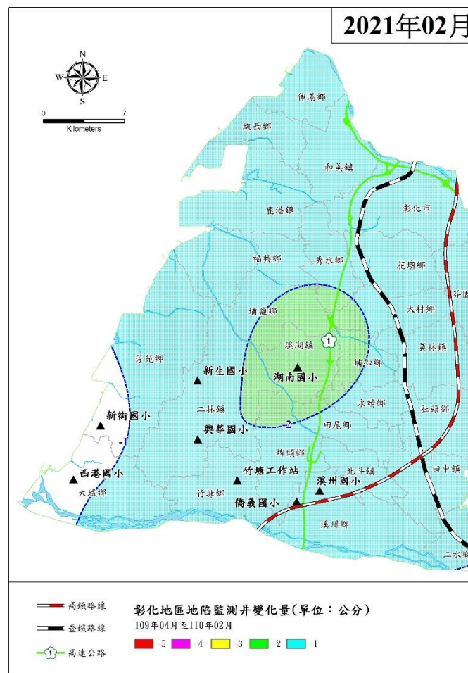
圖 1 彰化地區 109 年 4 月~110 年 2 月地陷監測井累積變化量圖
