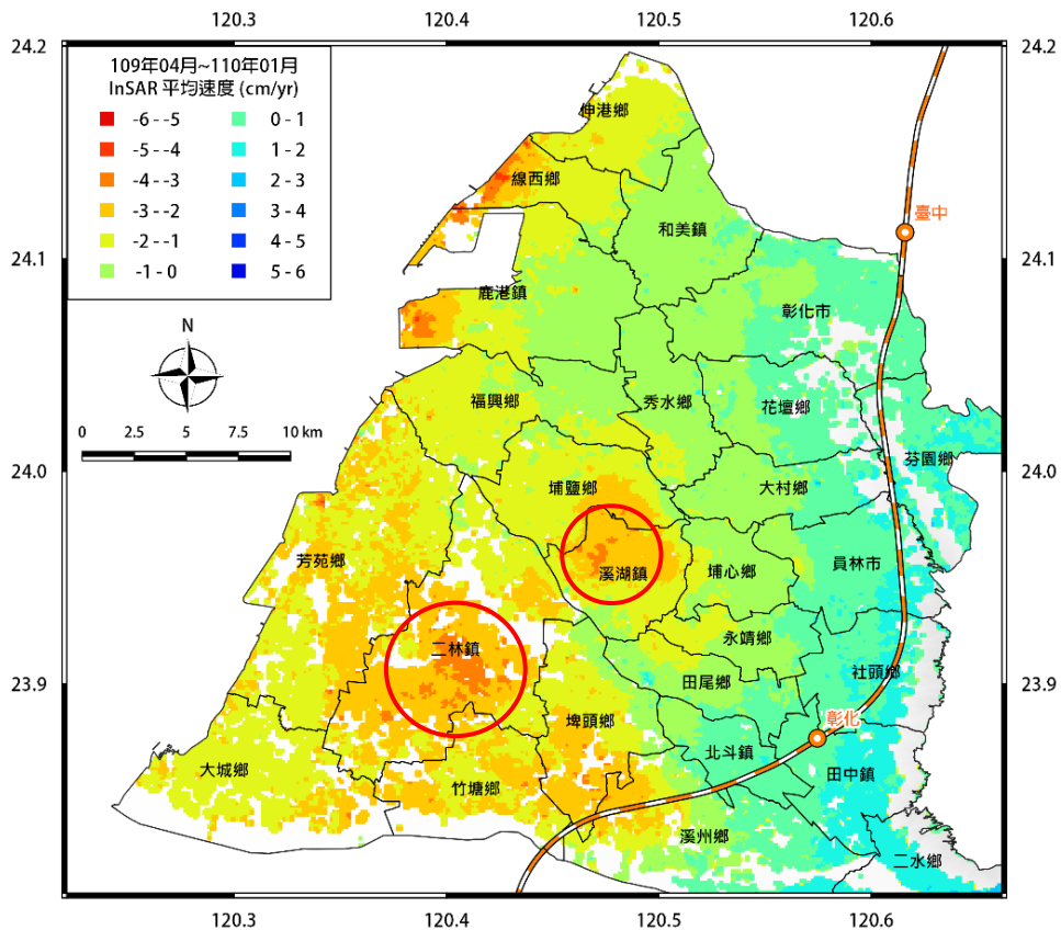
圖 23 彰化地區 109 年 4 月~110 年 1 月之平均位移速度場
