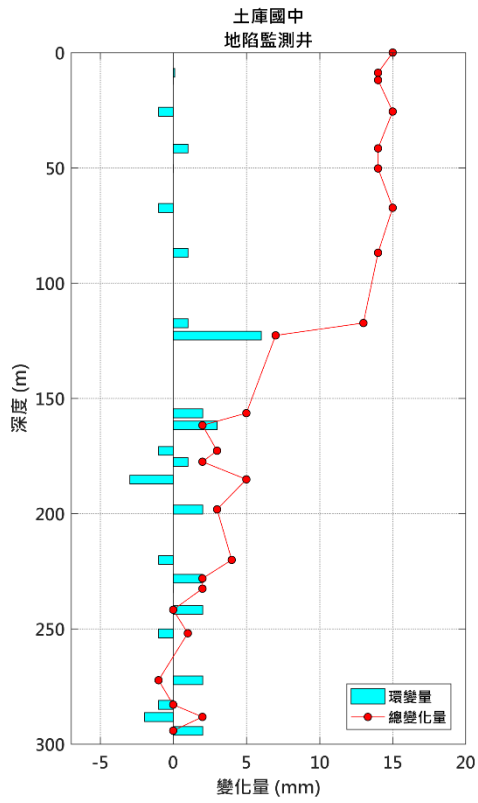
圖 6 土庫國中地陷監測井 2 月環變量分析圖
