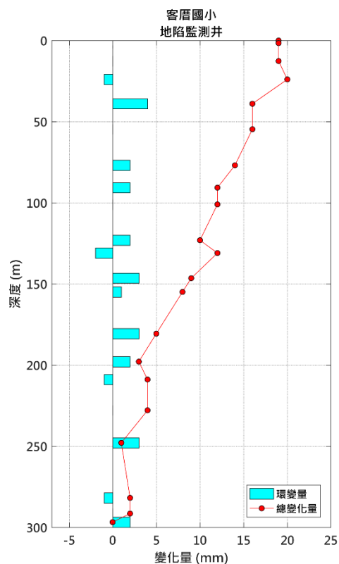
圖 14 客厝國小地陷監測井 2 月環變量分析圖
