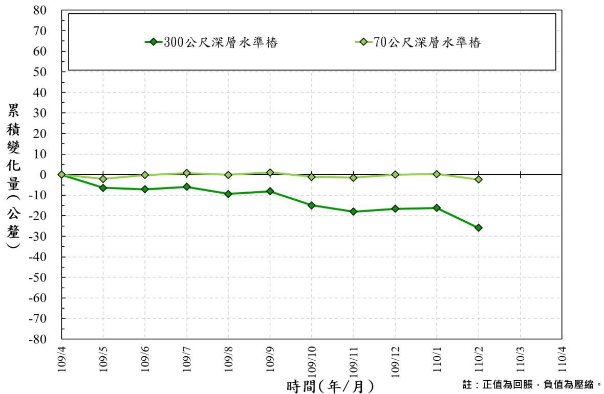
圖 21 雲林縣中科虎尾園區 109/4~110/2 監測成果比較圖
