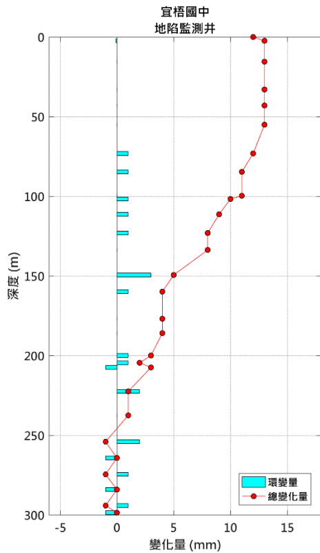
圖 12 宜梧國中地陷監測井 2 月環 變量分析圖
