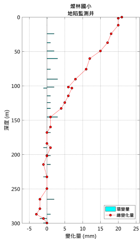
圖 16 水燦林國小地陷監測井 2 月環變量分析圖
