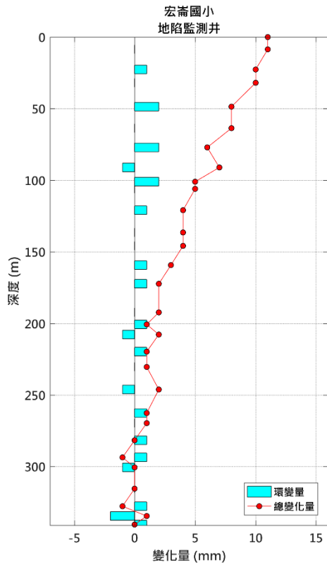
圖 10 宏崙國小地陷監測井 2 月環 變量分析圖
