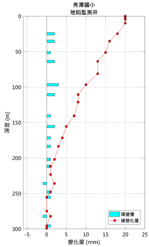
圖 11 秀潭國小地陷監測井 2 月環 變量分析圖
