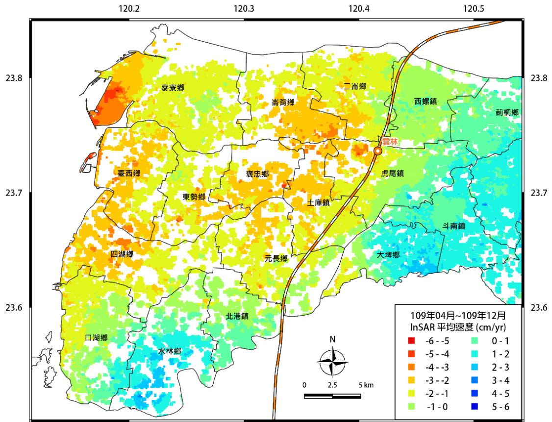
圖 24 雲林地區 109 年 4 月~109 年 12 月之平均位移速度場
