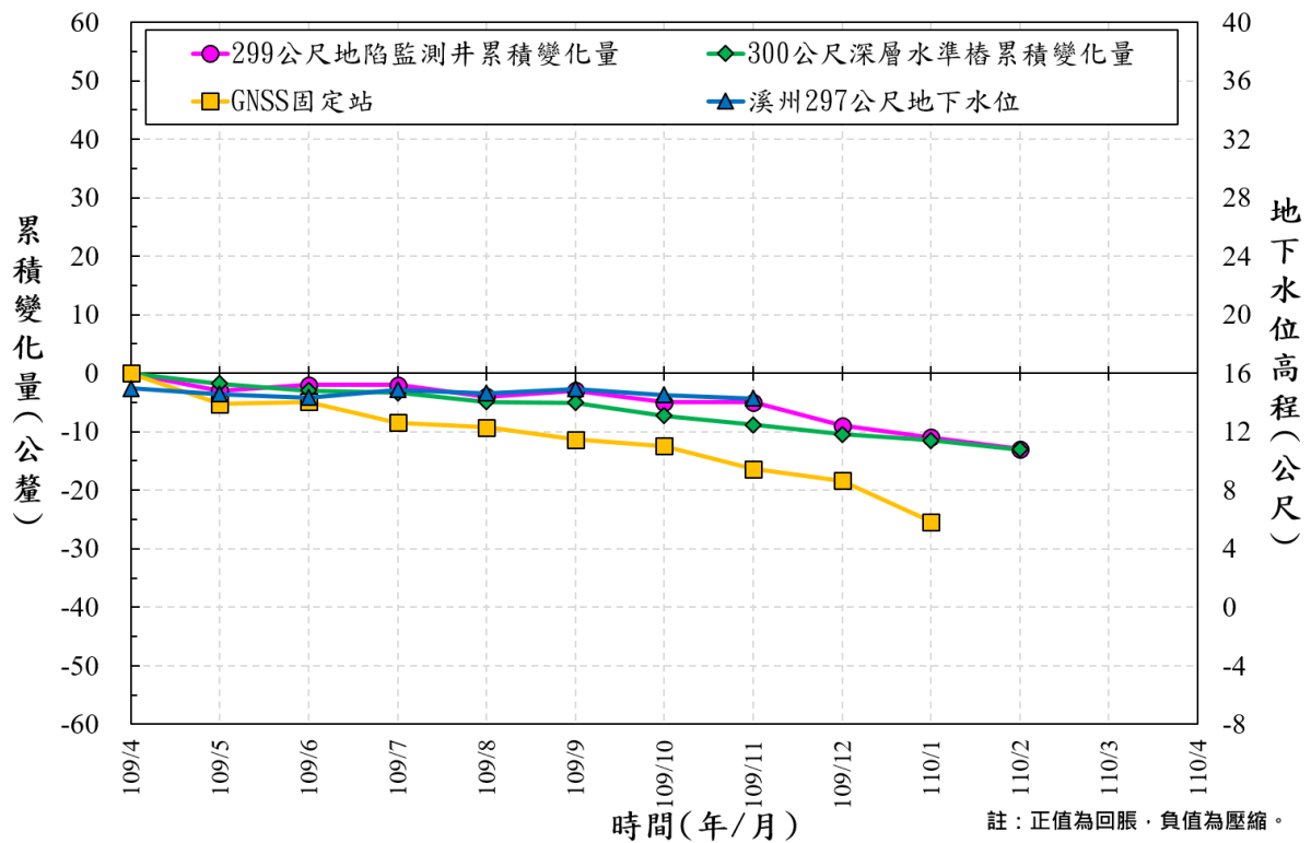
圖 18 彰化縣溪州國小 109/4~110/2 監測成果比較圖
