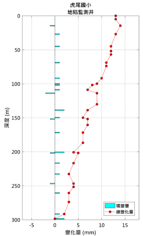
圖 13 虎尾國小地陷監測井 2 月環 變量分析圖
