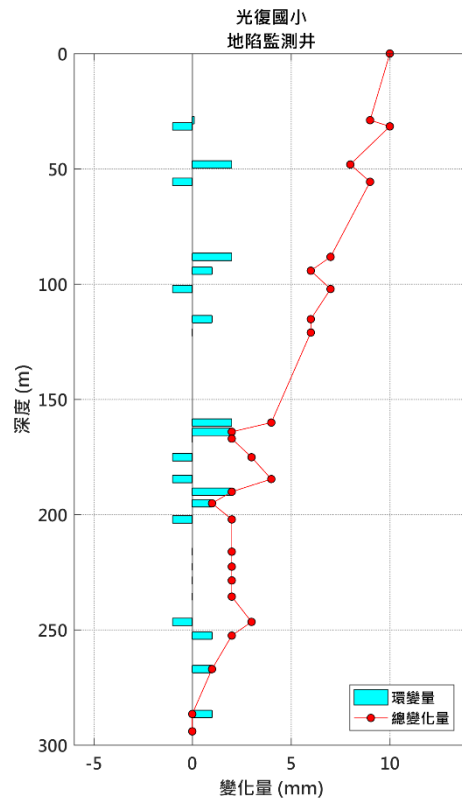
圖 9 光復國小地陷監測井 2 月環變量分析圖
