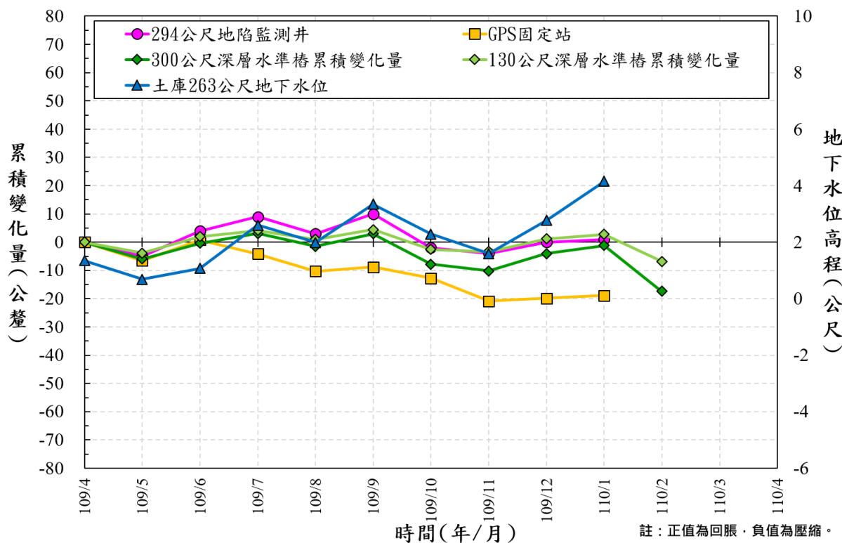
圖 19 雲林縣土庫國中 109/4~110/2 監測成果比較圖
