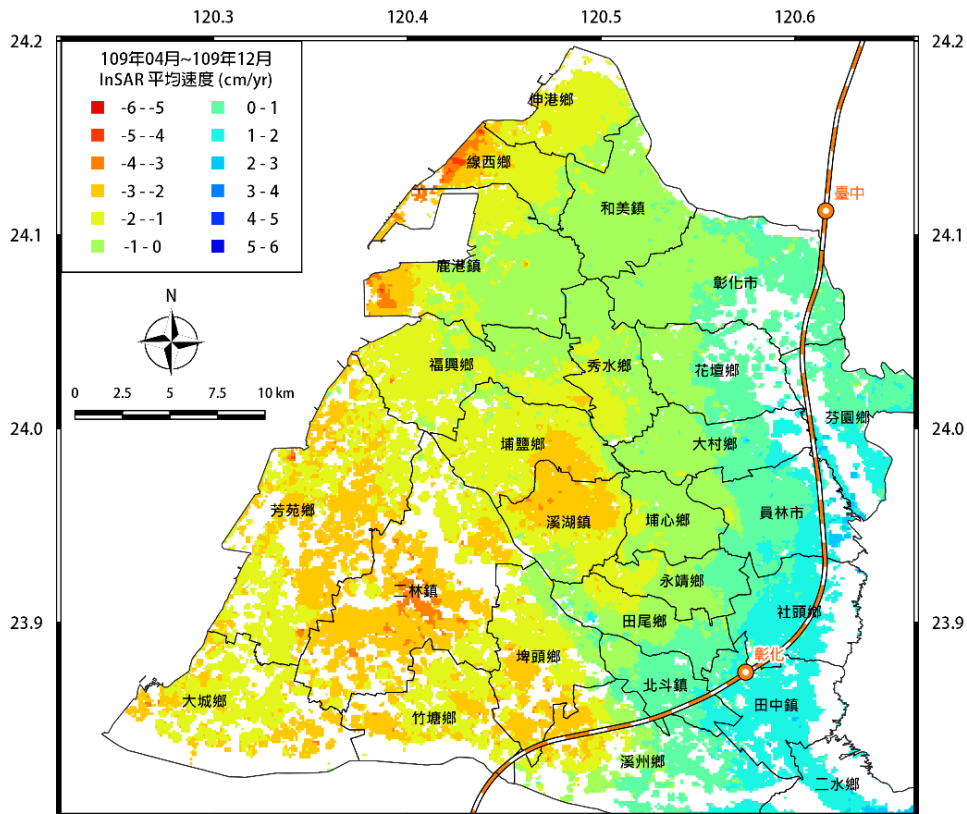
圖 22 彰化地區 109 年 4 月~109 年 12 月之平均位移速度場
