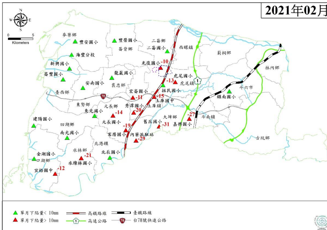
圖 5 雲林地區 110 年 2 月(單月)地陷監測井量測成果圖
