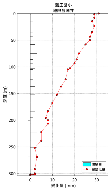
圖 17 舊庄國小地陷監測井 2 月環變量分析圖
