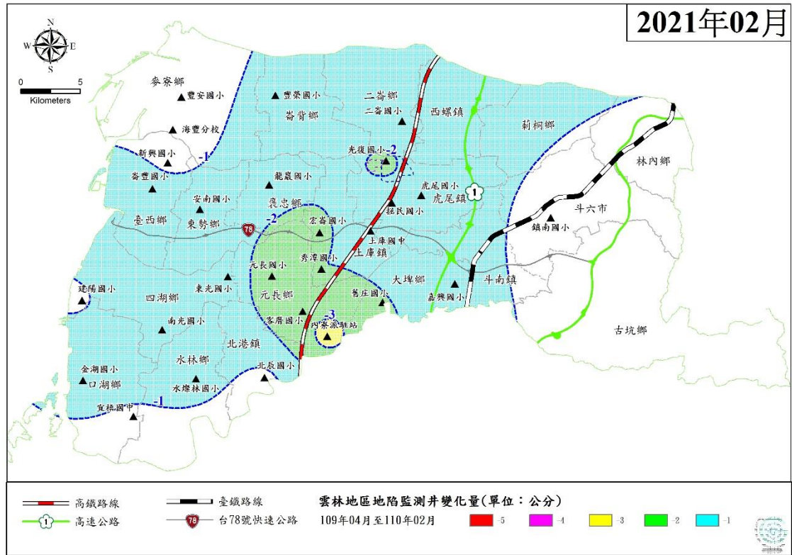
圖 2 雲林地區 109 年 4 月~110 年 2 月地陷監測井累積變化量圖 註：正值為回脹，負值為下陷。
