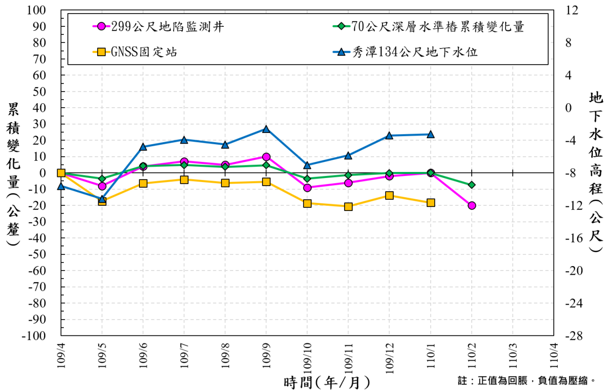
圖 20 雲林縣秀潭國小 109/4~110/2 監測成果比較圖
