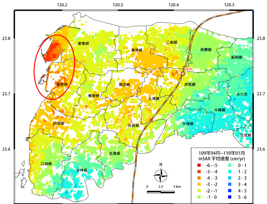
圖 25 雲林地區 109 年 4 月~110 年 1 月之平均位移速度場
