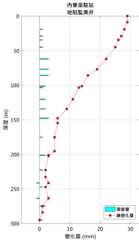
圖 8 內寮派駐站地陷監測井 2 月環變量分析圖
