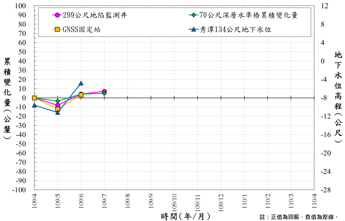
圖 10 雲林縣秀潭國小 109/4~109/7 監測成果比較圖
