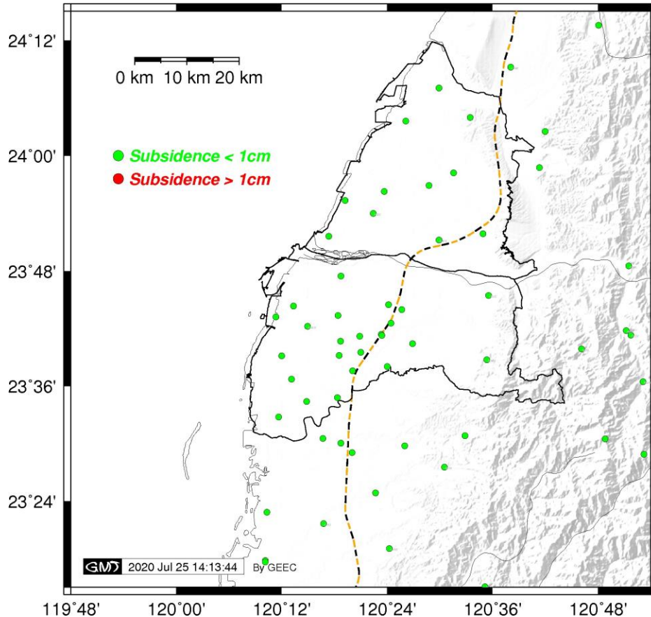
圖 6 彰雲地區 109 年 6 月 GNSS 固定站量測成果分析圖
