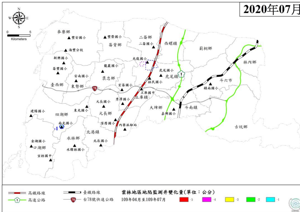
圖 2 雲林地區 109 年 4 月~109 年 7 月地陷監測井累積變化量圖
