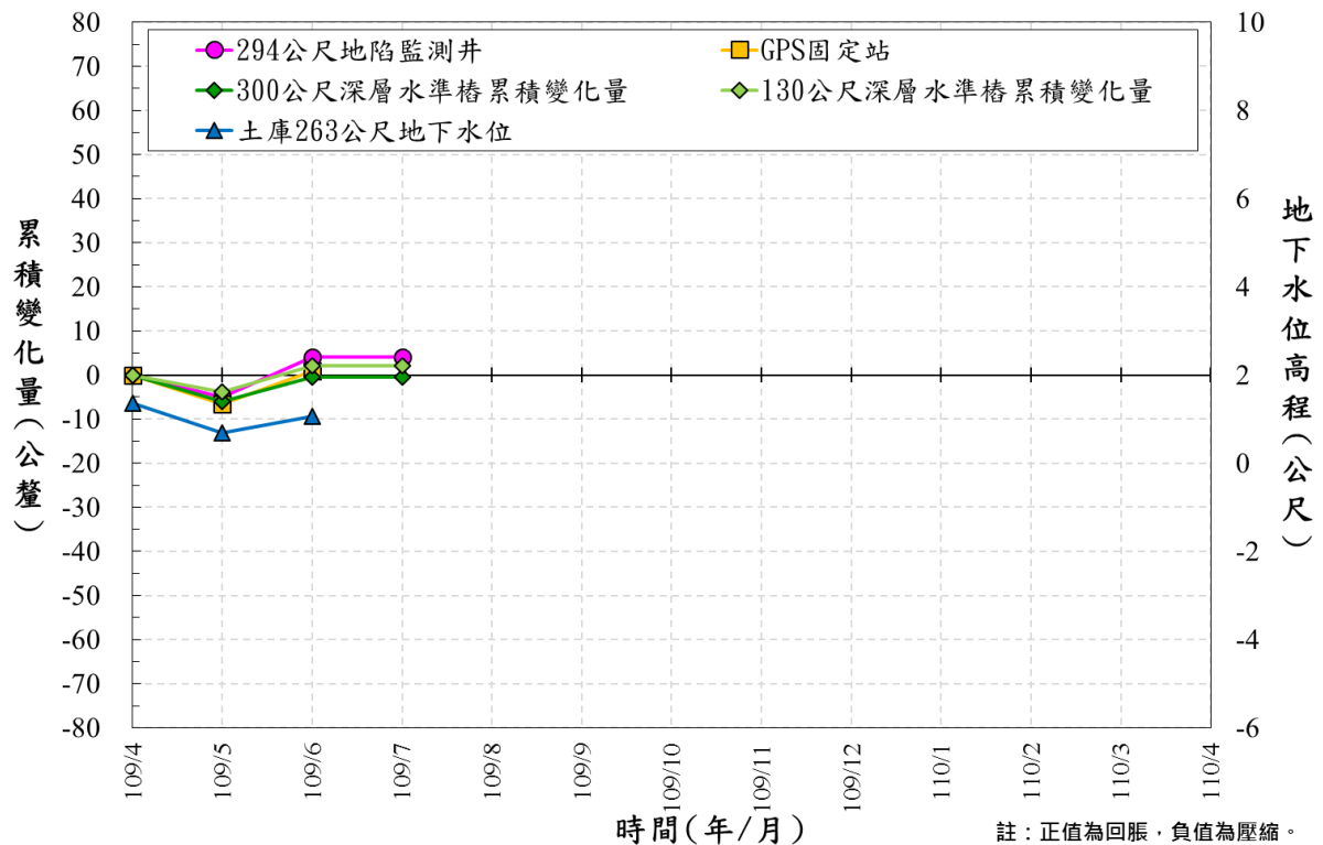
圖 9 雲林縣土庫國中 109/4~109/7 監測成果比較圖
