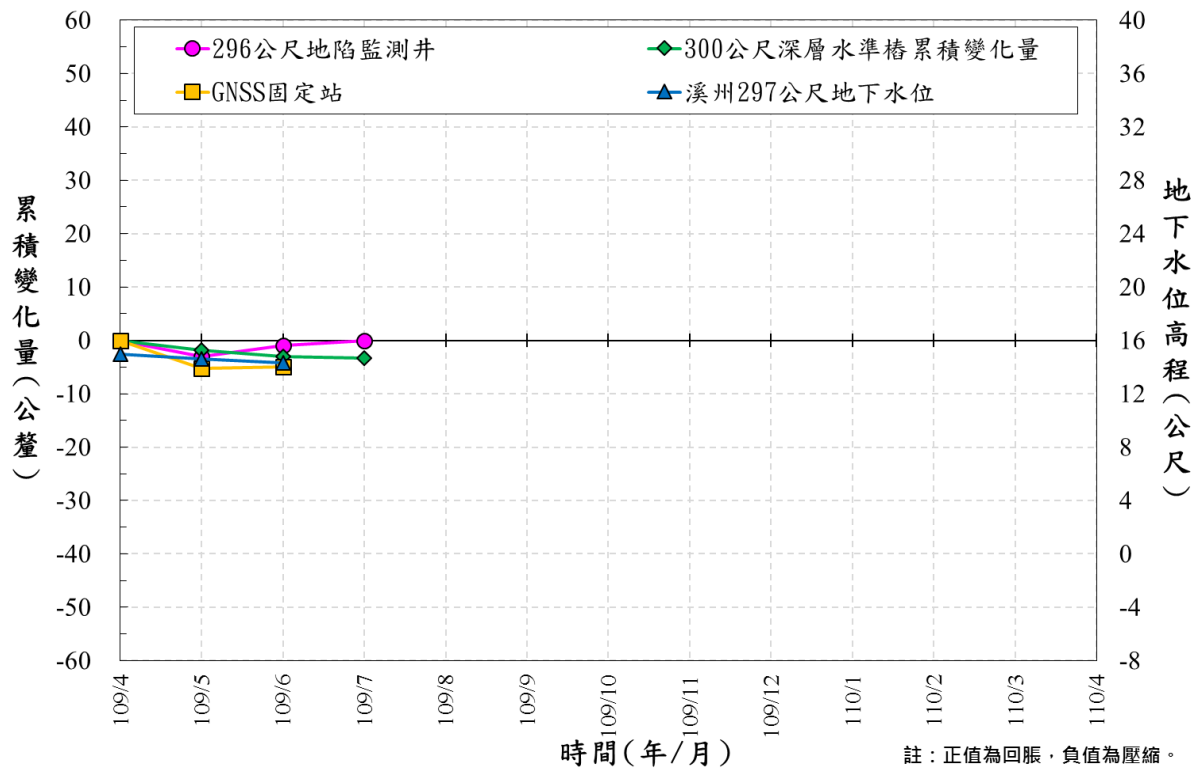
圖 8 彰化縣溪州國小 109/4~109/7 監測成果比較圖
