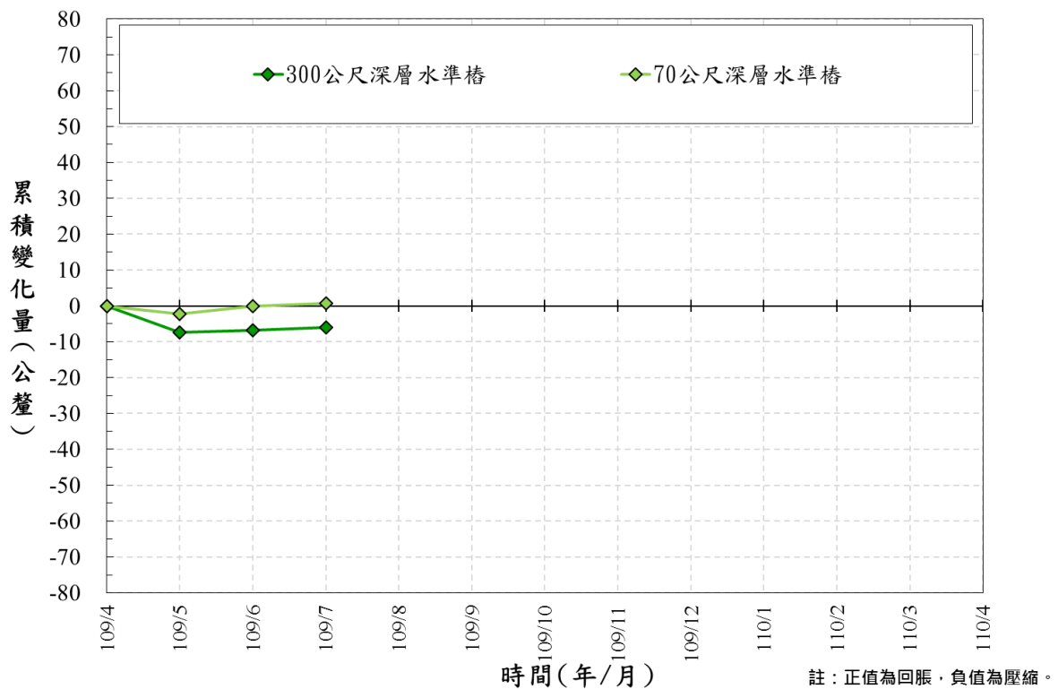
圖 11 雲林縣中科虎尾園區 109/4~109/7 監測成果比較圖
