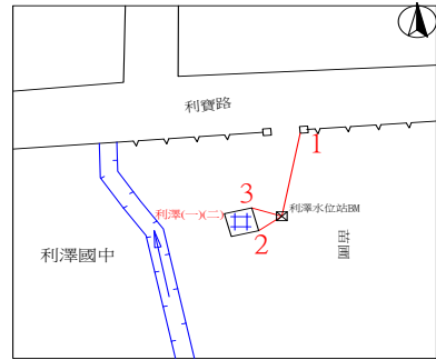
點位詳圖
