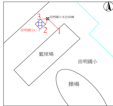
點位詳圖
