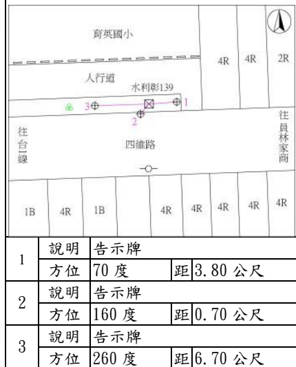
點位詳圖
