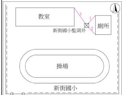
點位詳圖
