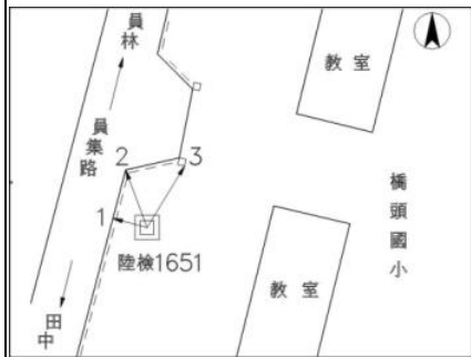
點位詳圖
