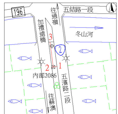
點位詳圖
