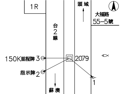
點位詳圖
