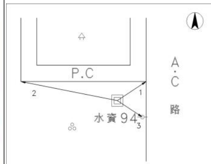
點位詳圖
