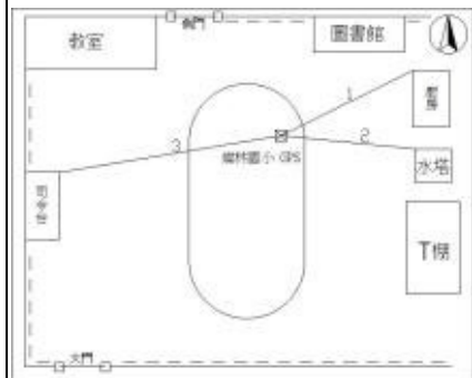
點位詳圖
